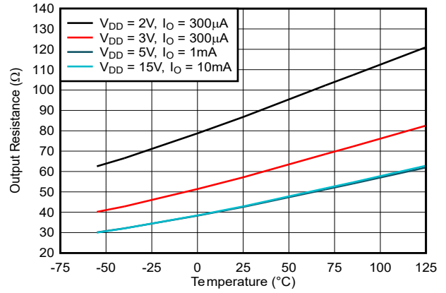
图 5-6. 输出高电阻与温度间的关系
