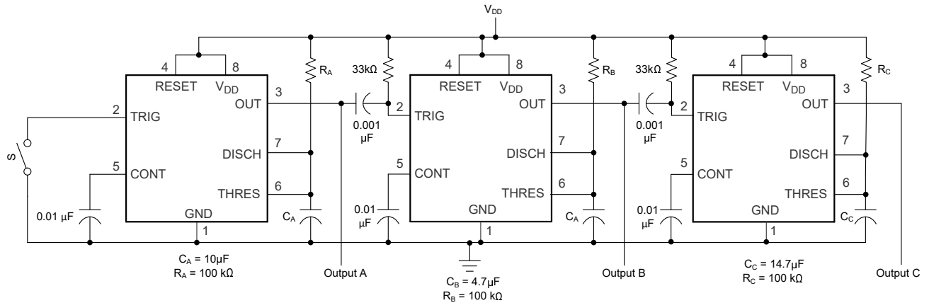
图 7-7. 顺序计时器电路
