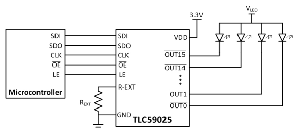
典型应用图
