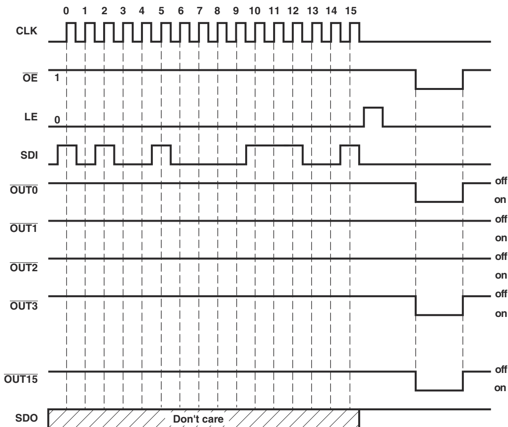
图 9-1. Timing Diagram
