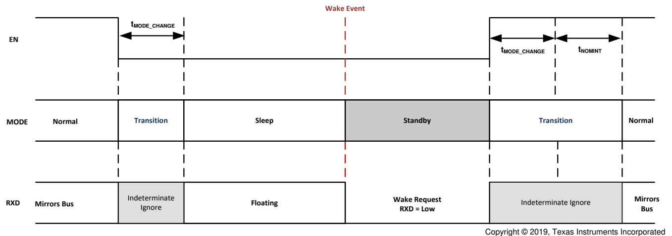
图 8-15. Mode Transitions
