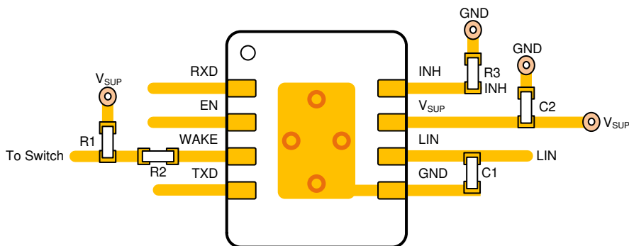
图 10-4. Layout Example
