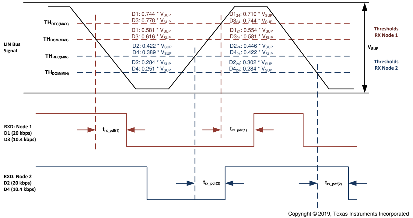
图 8-14. Propagation Delay
