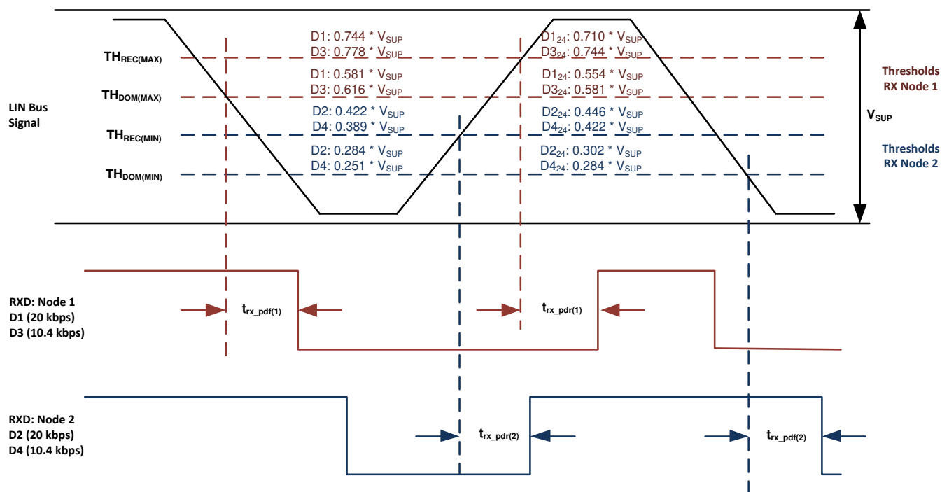
图 8-11. Propagation Delay
