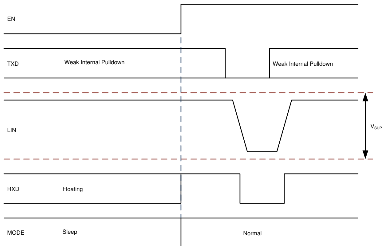
图 8-12. Mode Transitions
