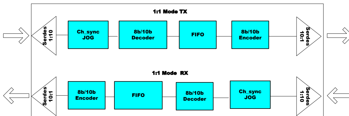
Figure 3-6. 1:1 Mode Datapath
