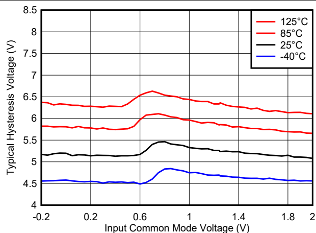
图 8-22. 迟滞电压与共模间的关系, 1.8V
