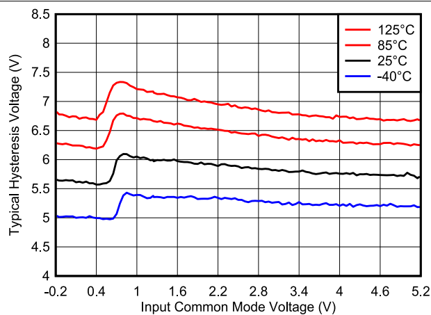
图 8-24. 迟滞电压与共模间的关系, 5V
