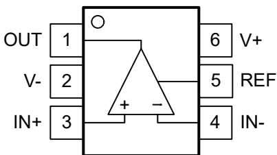
图 5-1. DCK , DBV 封装 6 引脚 SC-70、SOT-23 顶视图
