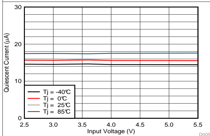
图 3. Quiescent Current
