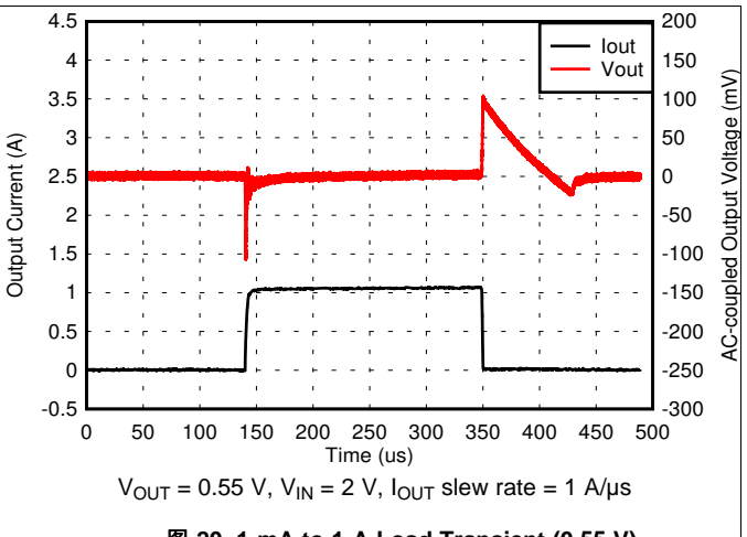
图 20. 1-mA to 1-A Load Transient (0.55 V)
