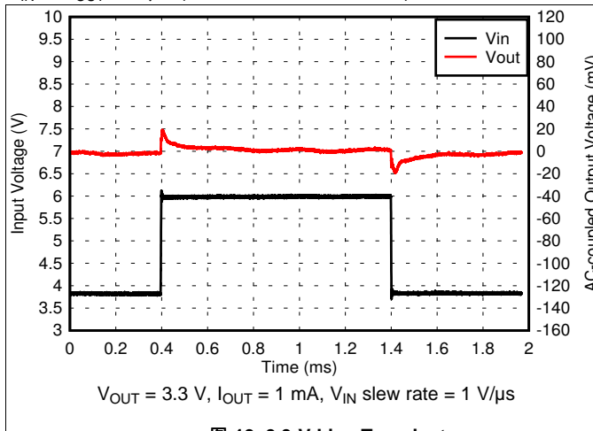
图 19. 3.3-V Line Transient
