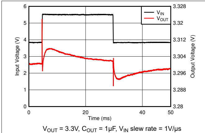
图 5-7. Line Transient
