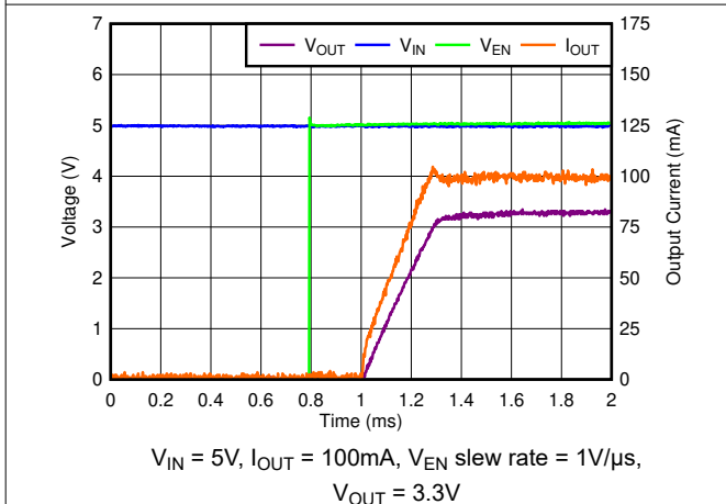
图 5-11. EN Start-Up
