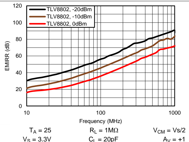
Figure 36. EMIRR 性能
