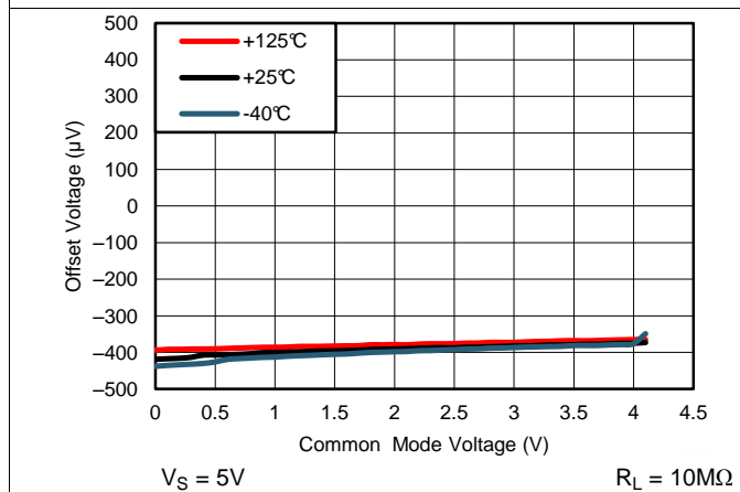
Figure 5. 典型偏移电压与共模电压间的关系
