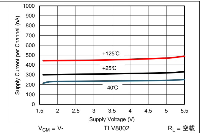
Figure 2. 电源电流与电源电压间的关系，TLV8802
