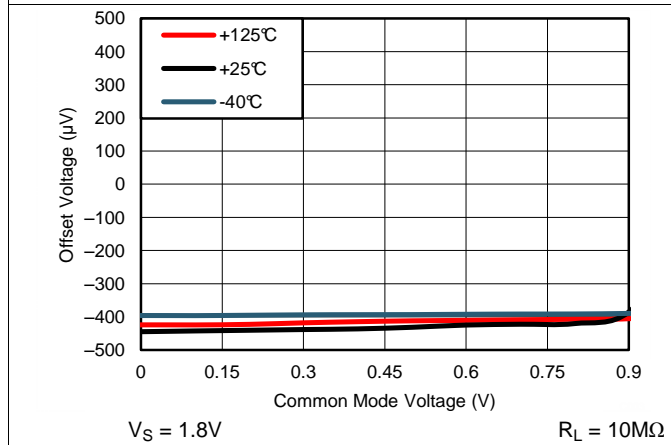
Figure 3. 典型偏移电压与共模电压间的关系
