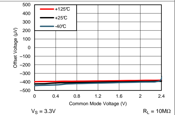
Figure 4. 典型偏移电压与共模电压间的关系
