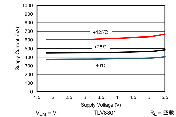
Figure 1. 电源电流与电源电压间的关系，TLV8801
