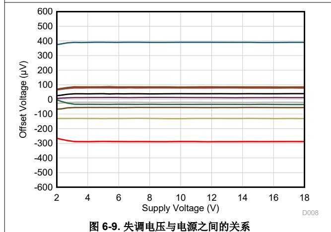
图 6-9. 失调电压与电源之间的关系
