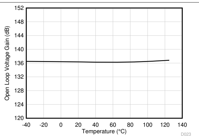
图 6-24. 开环电压增益与温度间的关系 (dB)
