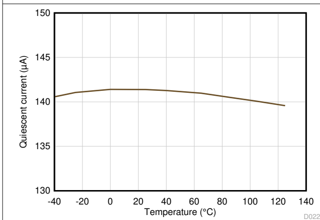
图 6-23. 静态电流与温度间的关系
