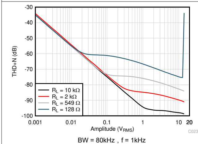
图 6-21. THD+N 与输出幅度间的关系
