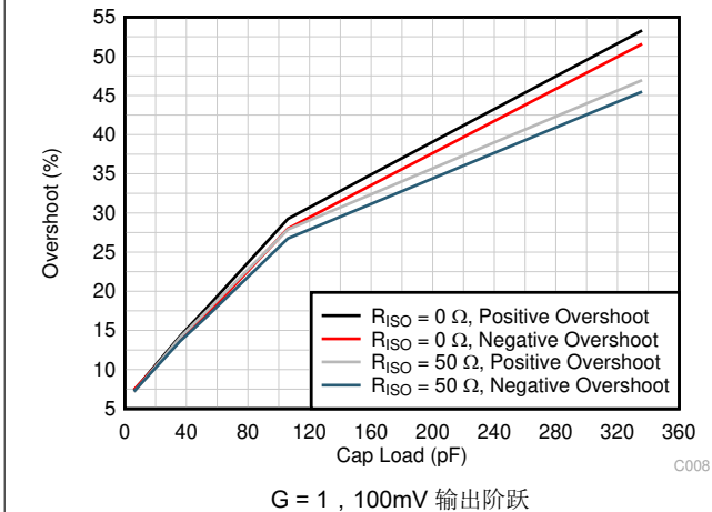
图 6-27. 小信号过冲与容性负载间的关系
