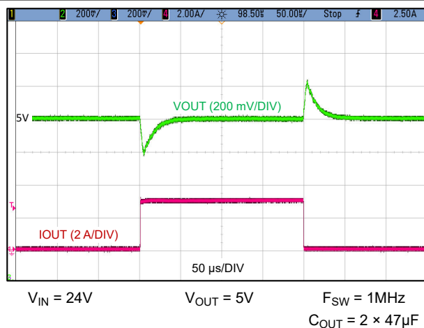
图 8-4. 负载瞬态 (0A 至 3A, 1A/μs)
