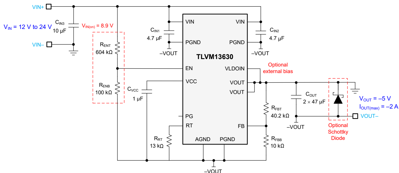
图 8-12. 电路原理图
