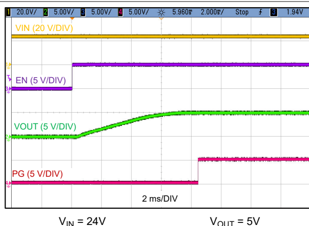
图 8-2. 启动波形
