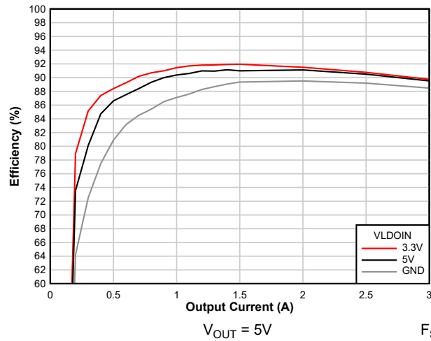
图 7-5. 通过 VLDOIN 实现的效率提升 (VOUT = 5V)
