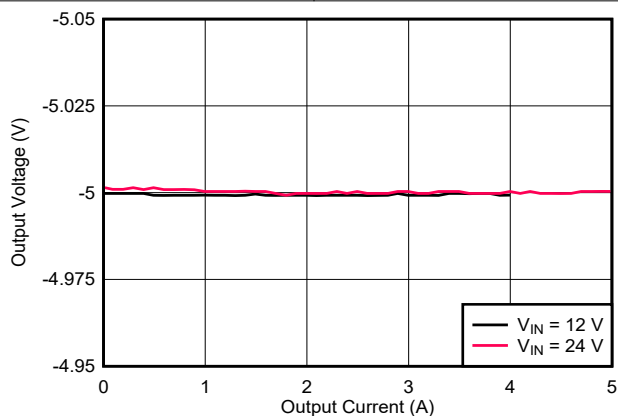
图 9-15. 负载调整率
