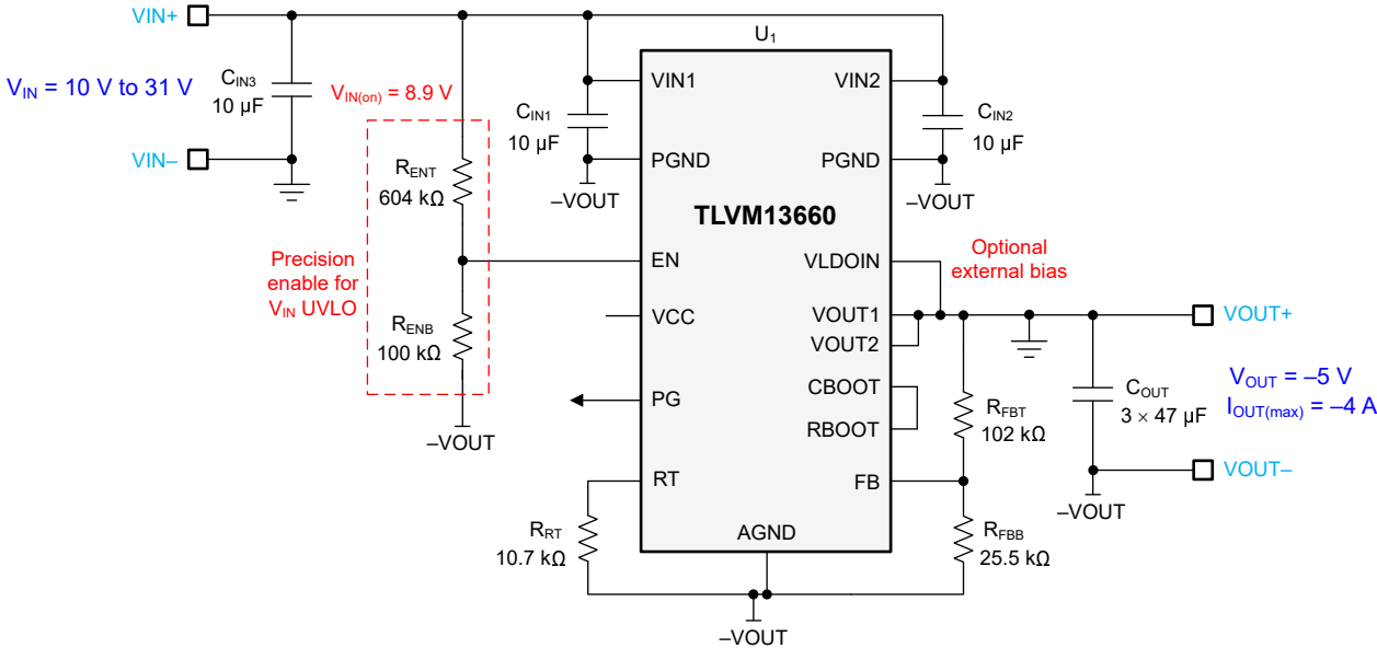
图 9-12. 电路原理图
