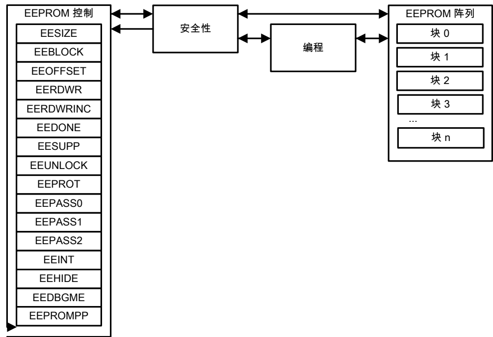
图 8-2. EEPROM 结构图
