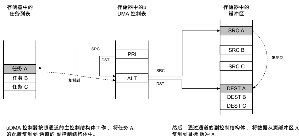
图 9-4. 存储器散聚模式：μDMA 复制序列
