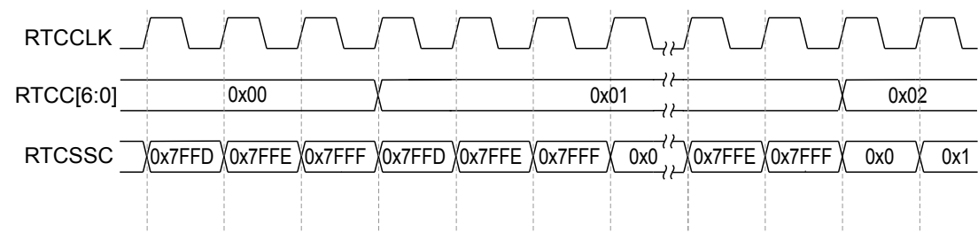
图 7-5. TRIM 值为 0x8002 时的计数器行为
