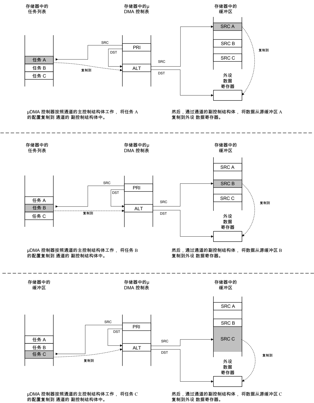
图 9-6. 外设散聚模式：μDMA 复制序列
