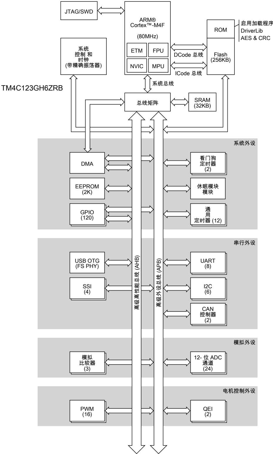
图 1-1. Tiva™ TM4C123GH6ZRB 微控制器高级框图
