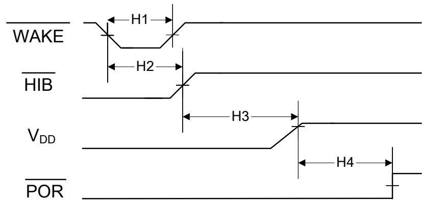
图 24-15. Hibernation Module Timing
