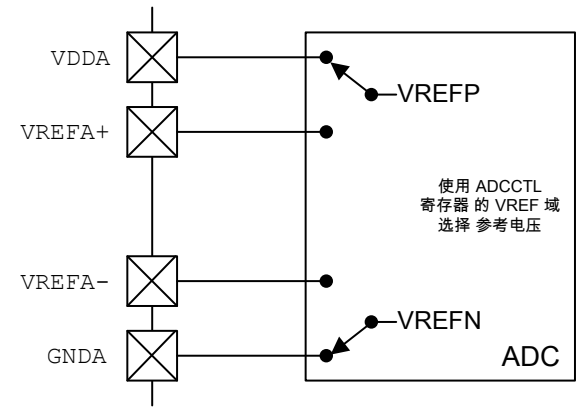
图 13-8. ADC 参考电压
