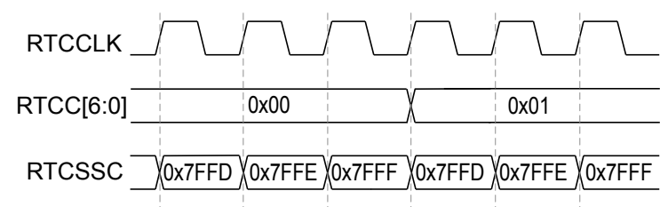
图 7-6. TRIM 值为 0x7FFC 时的计数器行为
