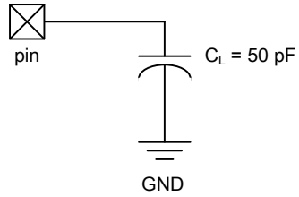
图 24-1. Load Conditions
