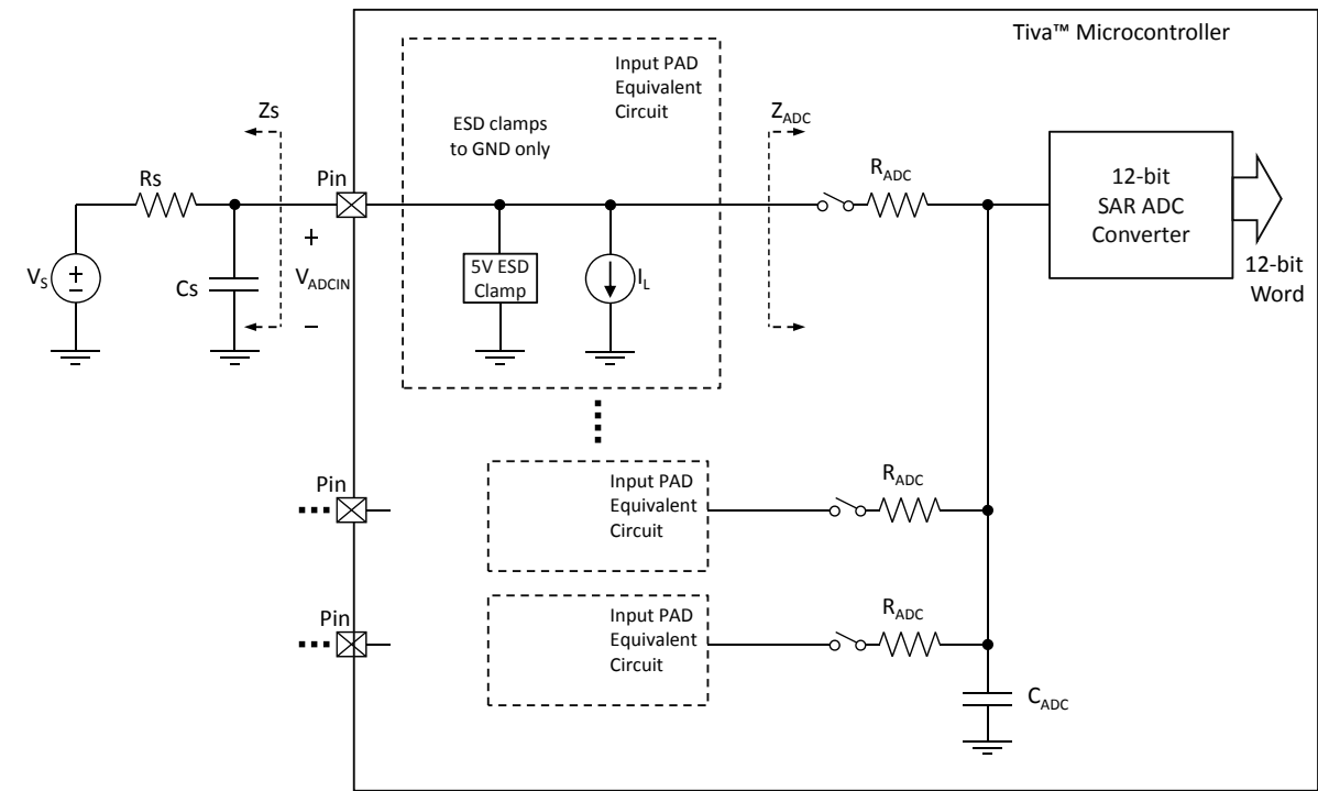
图 13-7. ADC 输入端等效框图
