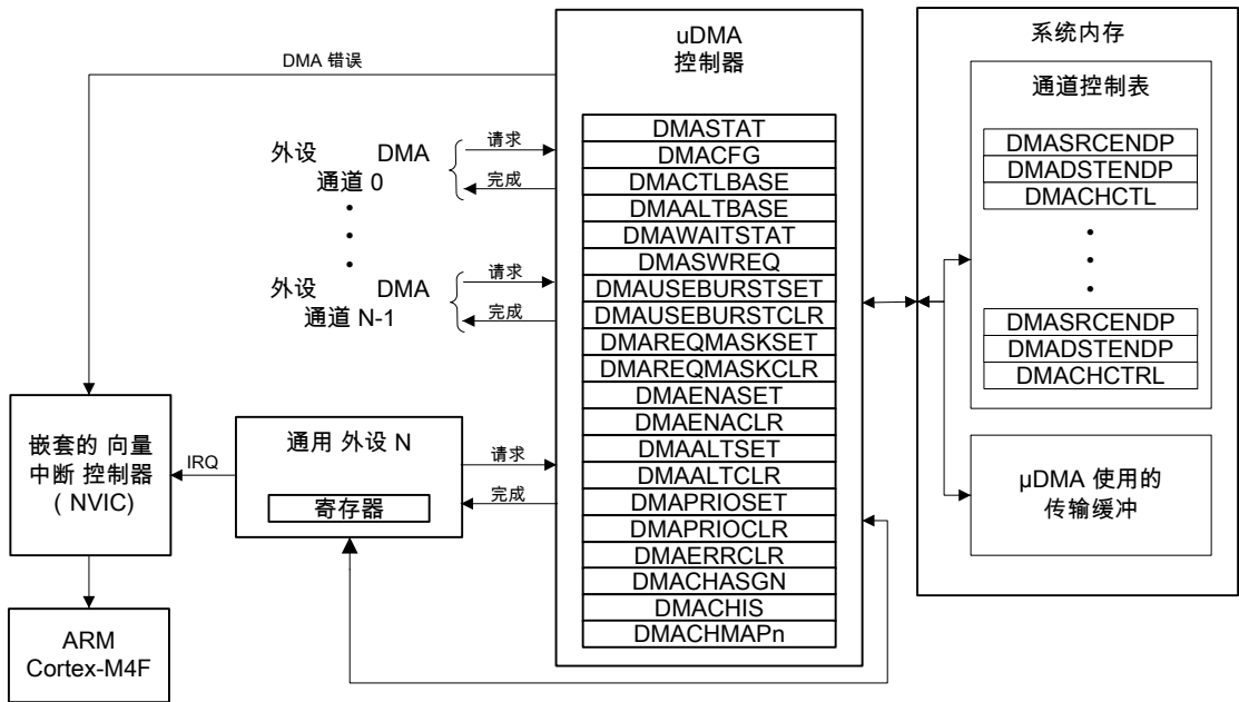
图 9-1. μDMA 结构图
