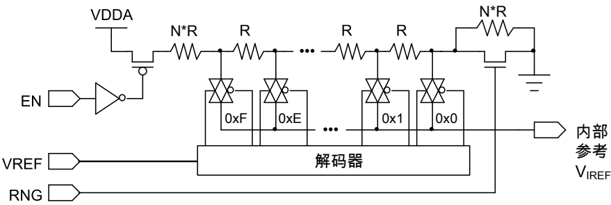
图 19-3. 比较器内部参考结构
