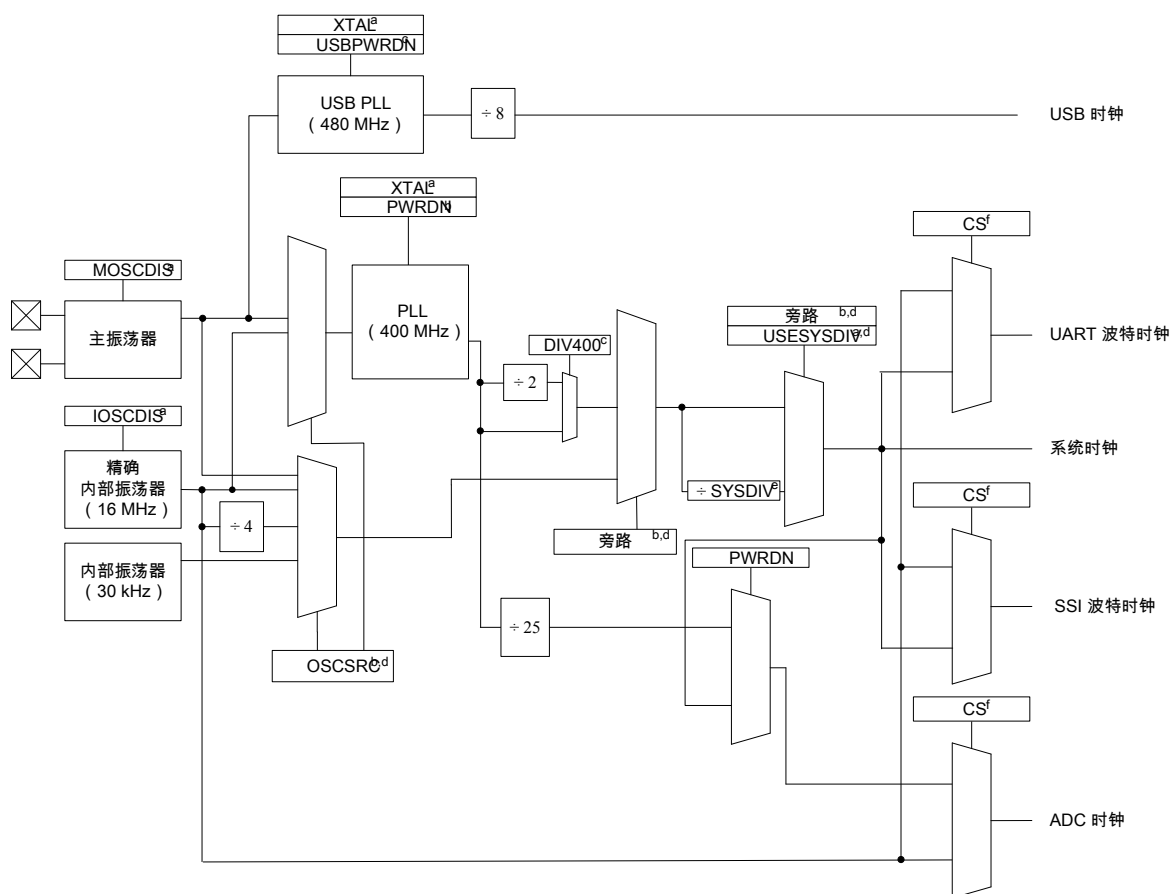
图 5-5. 主时钟树
