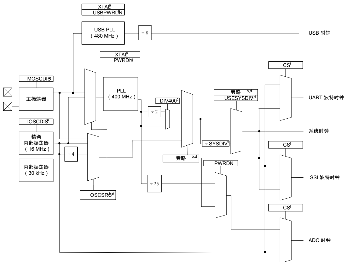
图 5-5. 主时钟树
