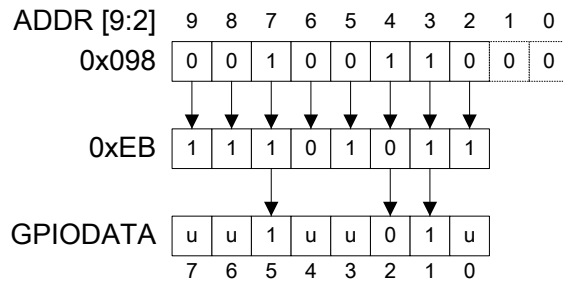
图 9-3. GPIODATA 写实例
