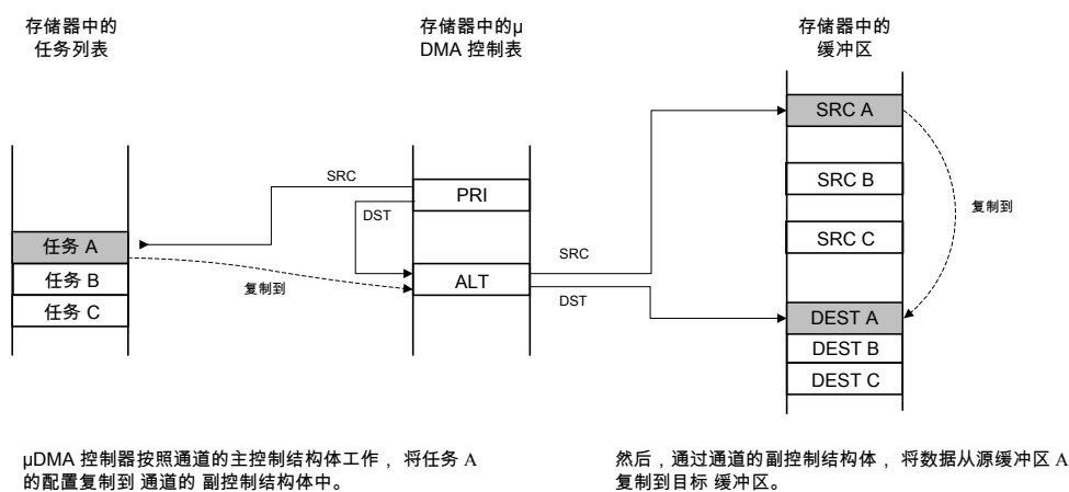
图 8-4. 存储器散聚模式：μDMA 复制序列
