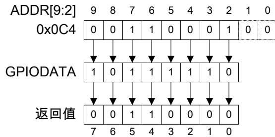
图 9-4. GPIODATA 读实例
