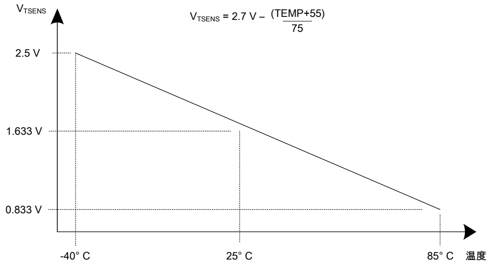
图 12-11. 内部温度传感器特性
