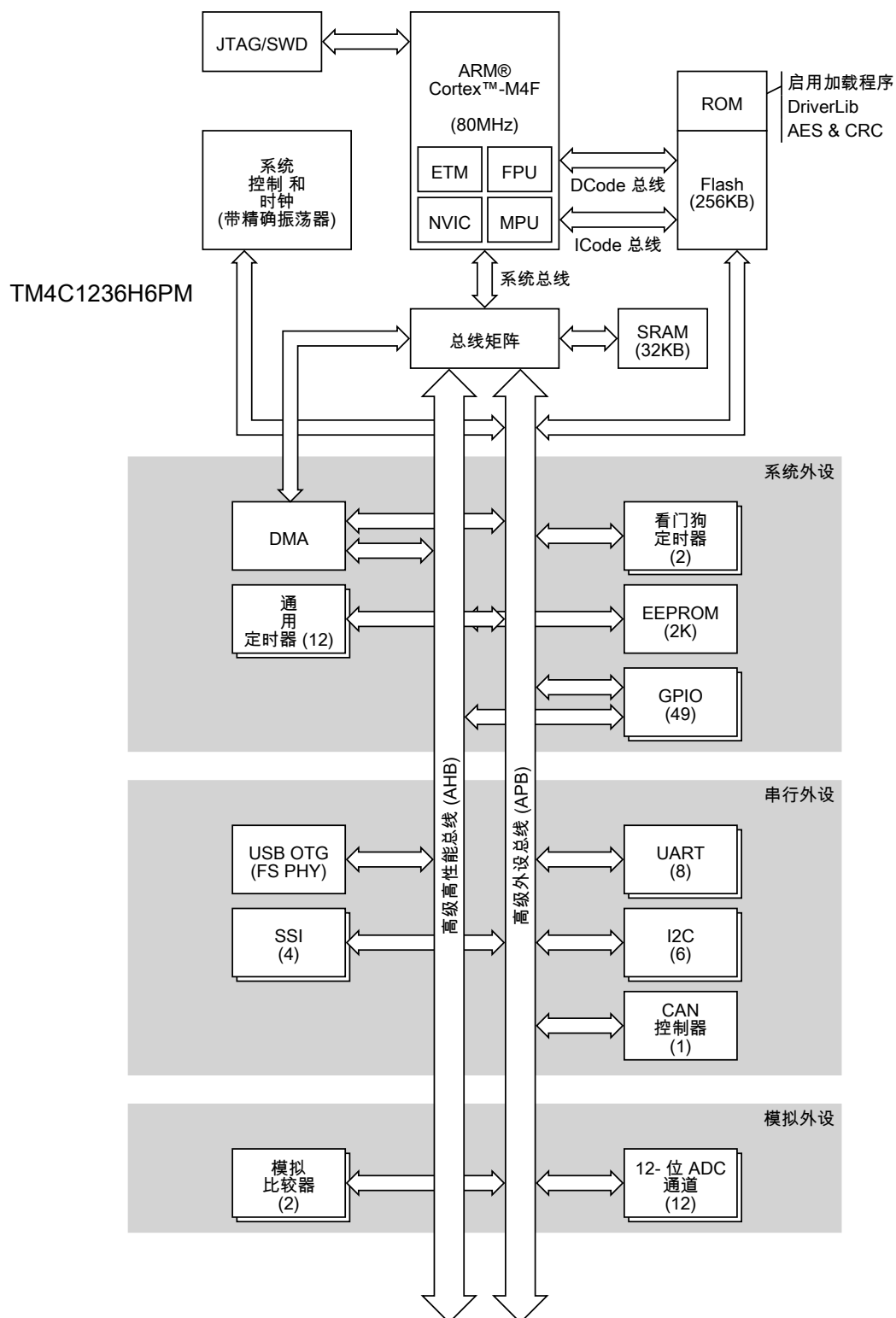
图 1-1. Tiva™ TM4C1236H6PM 微控制器高级框图
