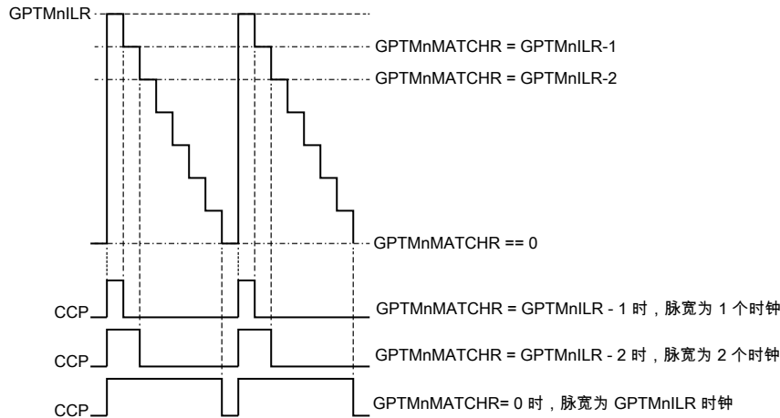
图 10-8. CCP 输出，GPTMTnILR &gt; GPTMTnMATCHR
