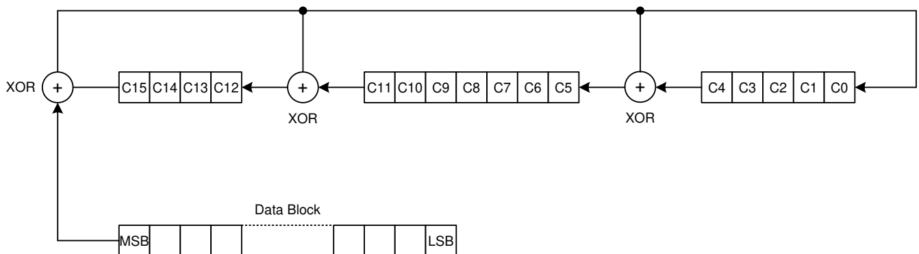
图 8-17. CRC 模块
