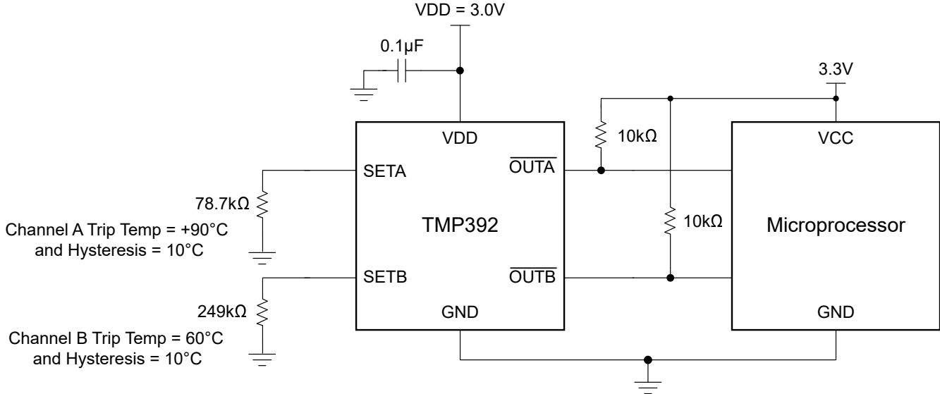
图 7-3. 阈值为 +90°C 和 +60°C 且迟滞为 10°C 的 TMP392 示例电路
