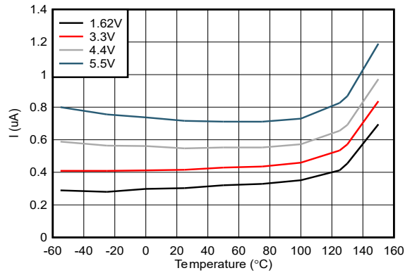
图 5-1. 平均电源电流与工作温度间的关系
