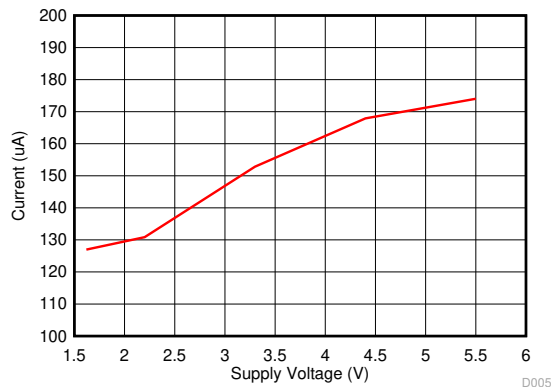
图 5-5. 转换电流与电源电压间的关系
