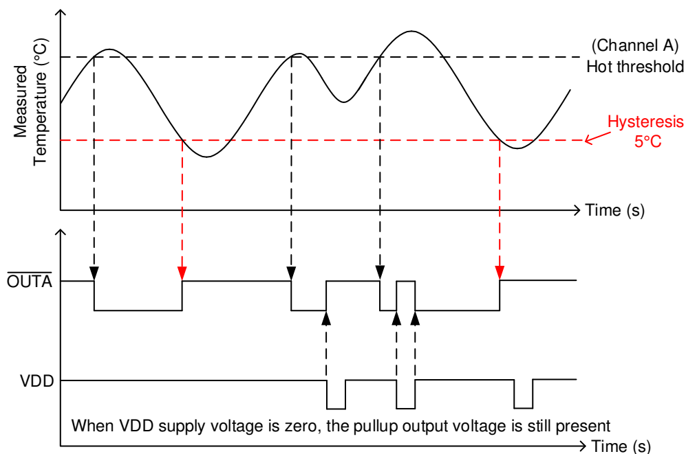
图 7-6. TMP392 单通道 (热) 运行阈值和迟滞
