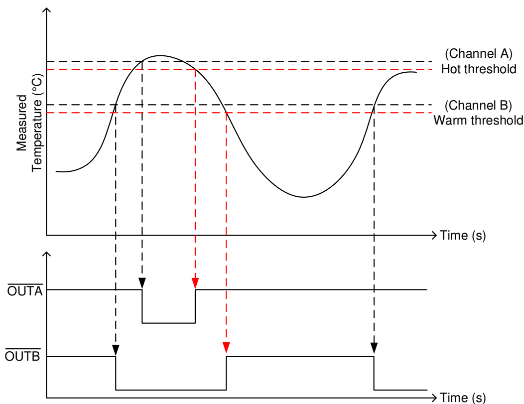
图 7-2. 具有热/温阈值和迟滞功能的 TMP392 输出
