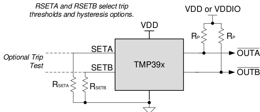
图 7-1. 简化原理图
