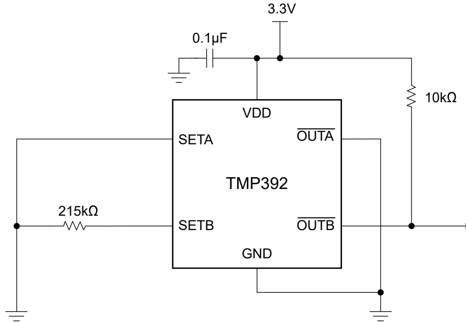
图 7-7. 具有 55°C 跳变点和 10°C 迟滞的 TMP392 单通道 (温) 运行示例电路
