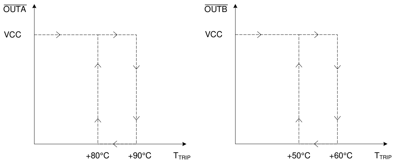
图 7-4. 具有迟滞功能的 TMP392 输出响应
