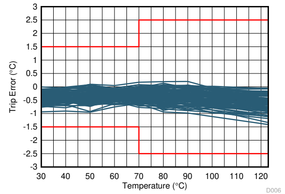
图 5-2. 热跳闸点精度与工作温度间的关系
