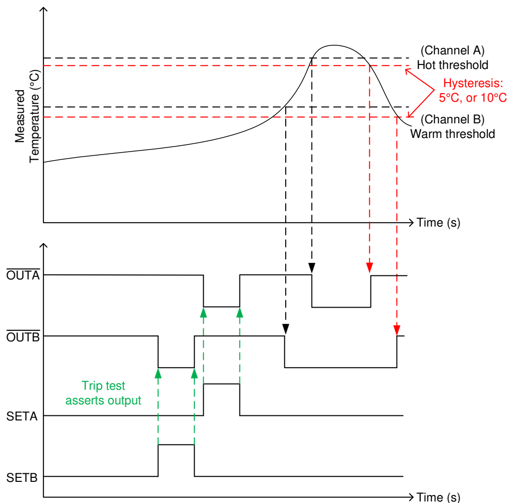
图 6-2. TMP392 跳闸测试操作
