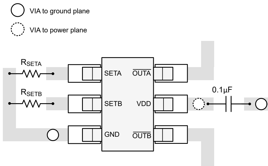
图 7-8. TMP392 建议布局
