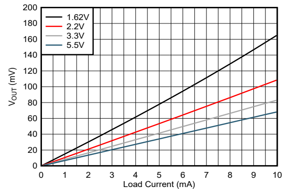
图 5-6. 输出电压与负载电流间的关系
