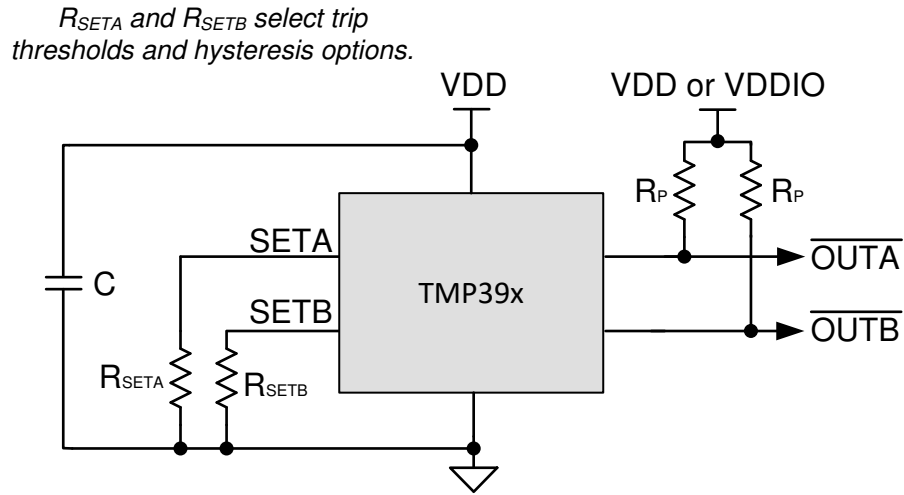
图 6-1. 简化版原理图
