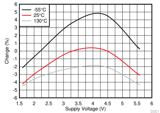
图 5-4. 采样周期变化与电源电压间的关系
