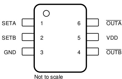
图 4-1. DRL 封装 6 引脚 SOT-563 顶视图
