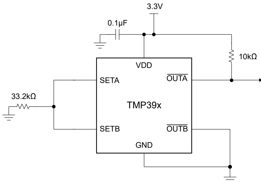
图 7-5. 具有 78°C 跳变点和 5°C 迟滞的 TMP392 单通道 (热) 运行示例电路
