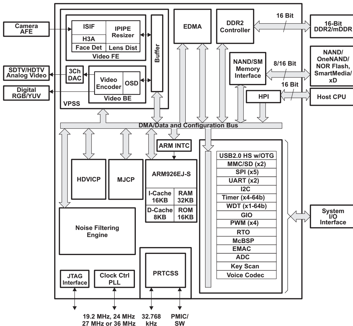
图 1-1. 功能方框图
