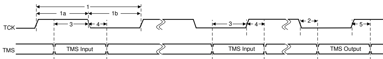
图 6-27. cJTAG 时序
