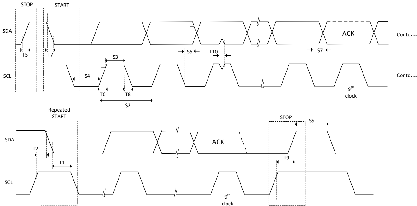
图 6-63. I2C 时序图
