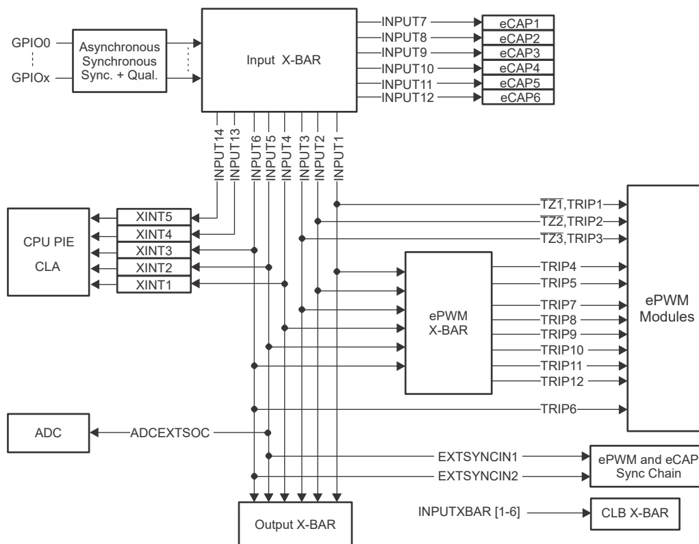
图 5-3. 输入 X-BAR
