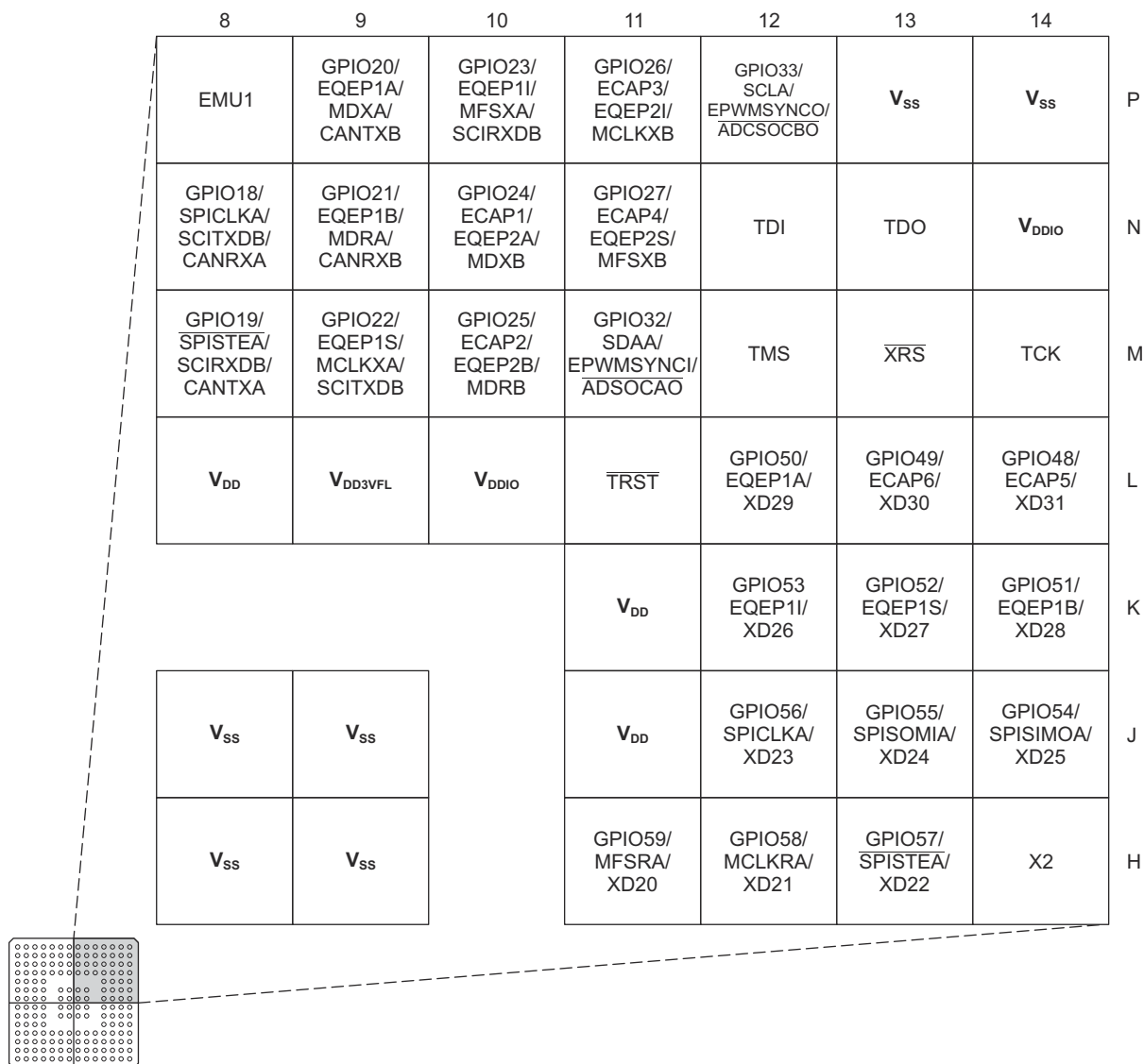
图 6-7. F2833x、F2823x 176 焊球 ZJZ 塑料 BGA (右上象限) (底视图)
