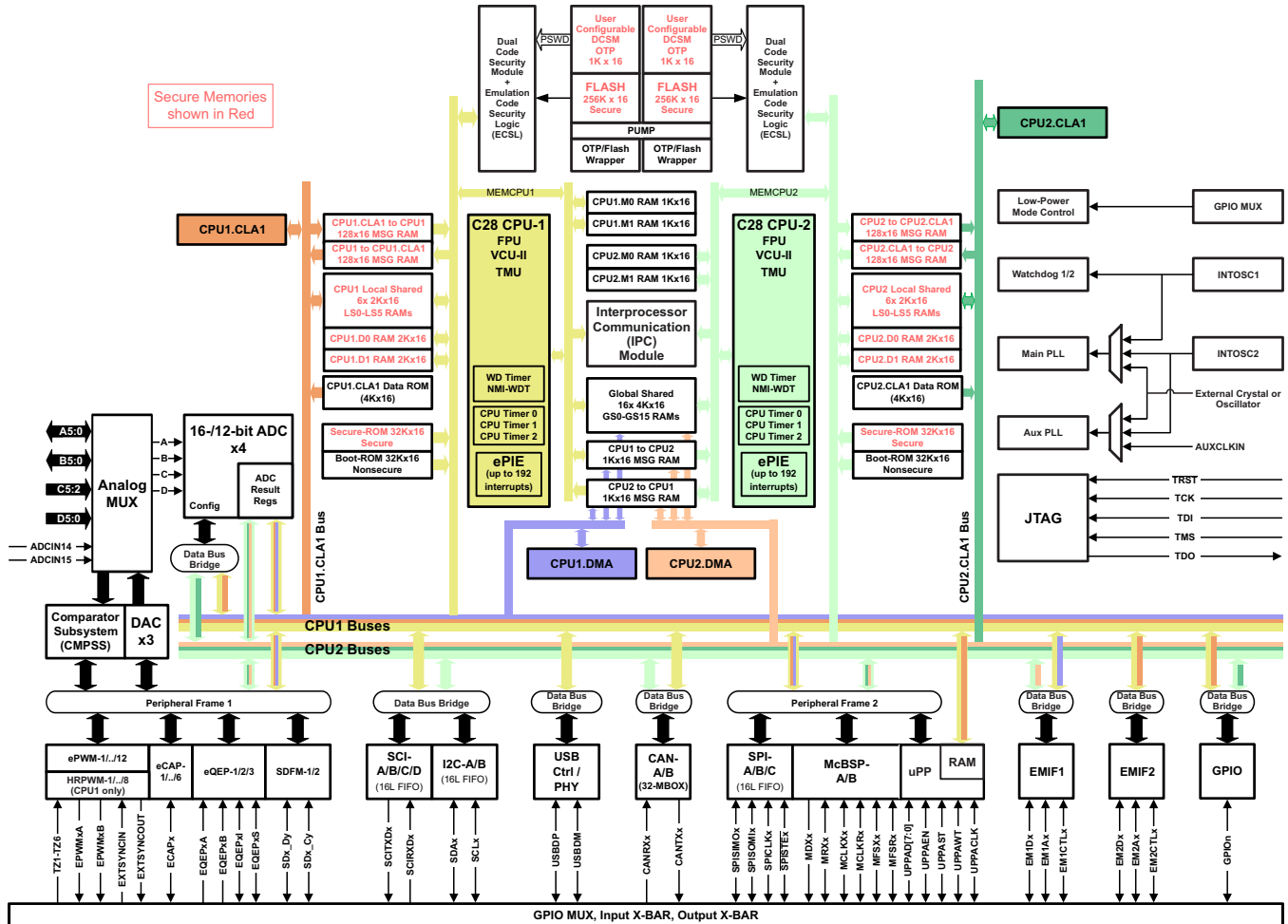
图 1-1. 功能框图
