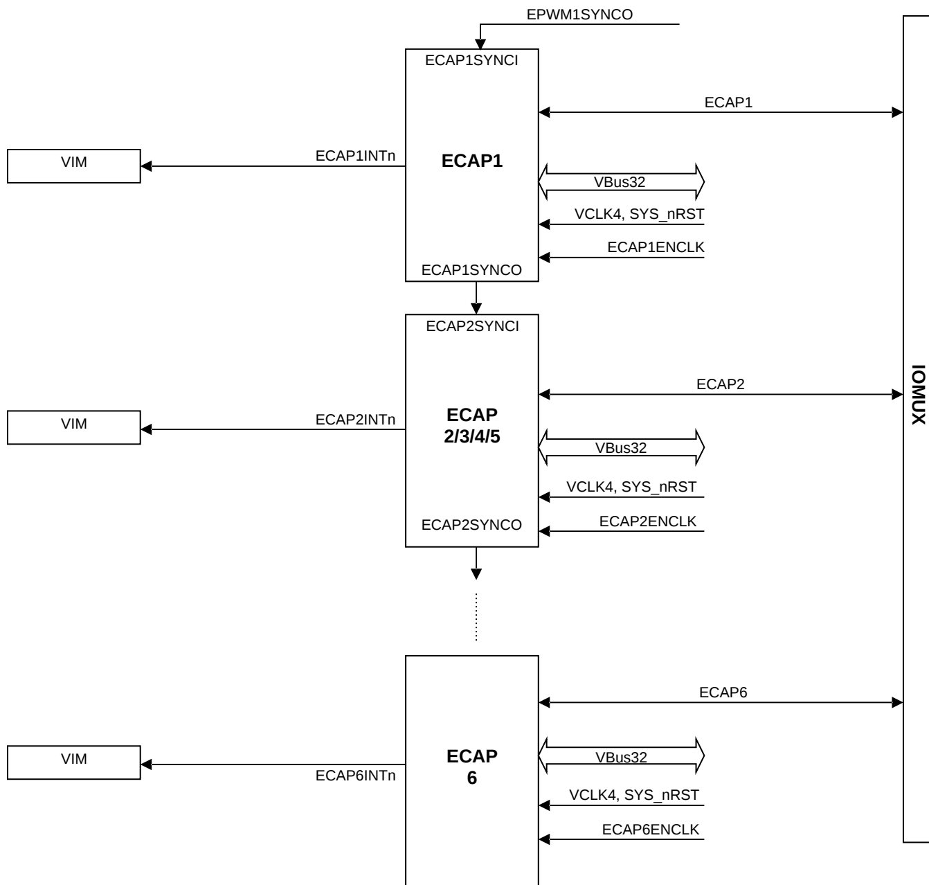
图 6-6. eCAPx Module Connections
