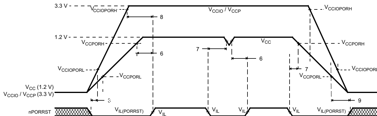
图 5-1. nPORRST Timing Diagram (A)
