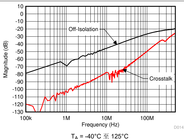
图 5-14. 串扰和关断隔离与频率之间的关系
