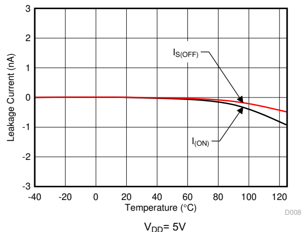
图 5-8. 泄漏电流与温度间的关系
