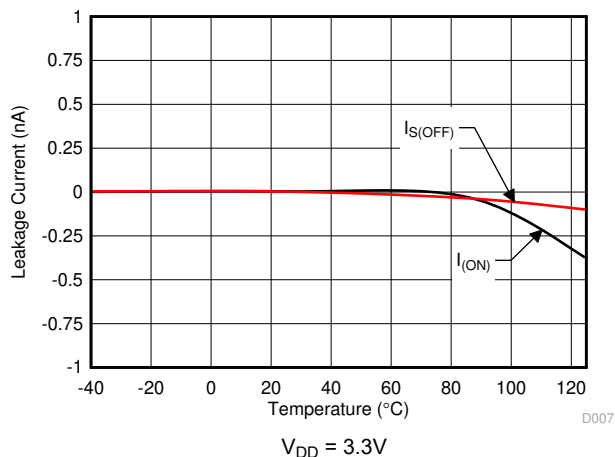
图 5-7. 泄漏电流与温度间的关系
