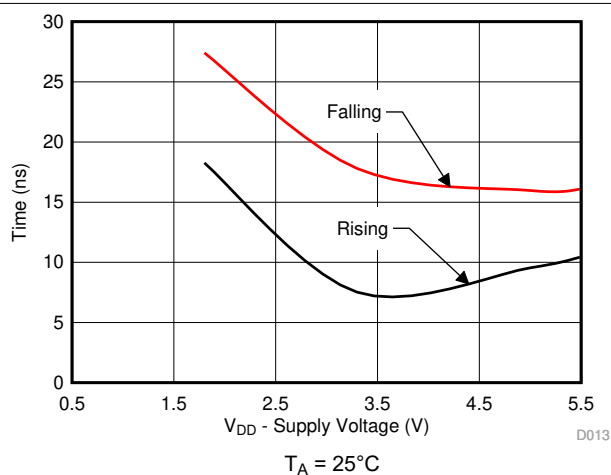
图 5-13. 输出 T_{\text{TRANSITION}} 与电源电压间的关系
