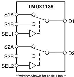
图 7-1. TMUX1136 功能方框图
