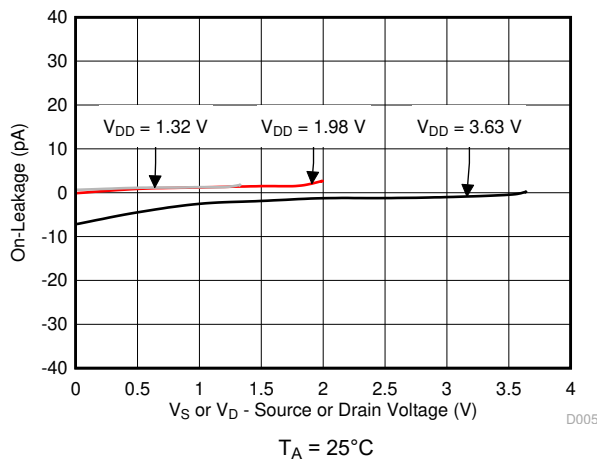
图 5-5. 导通漏电流与源极电压或漏极电压间的关系
