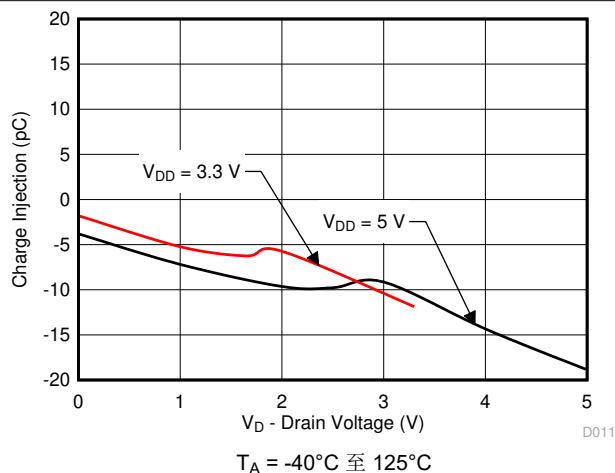
图 5-11. 电荷注入与漏极电压间的关系
