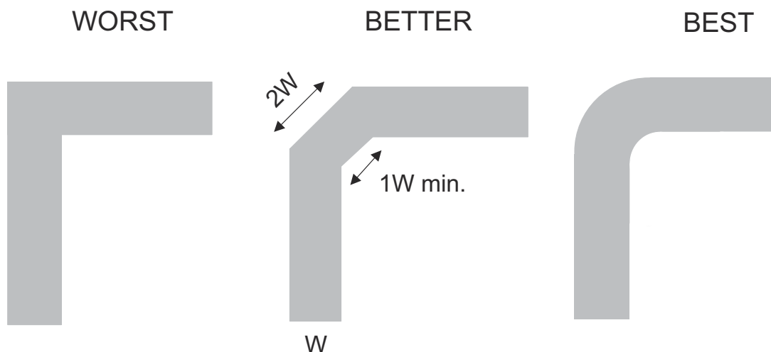
图 8-3. 布线示例
