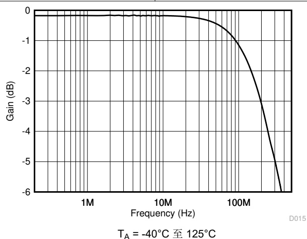
图 5-15. 导通响应与频率间的关系
