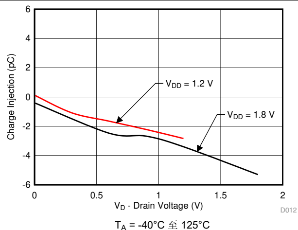
图 5-12. 电荷注入与漏极电压间的关系
