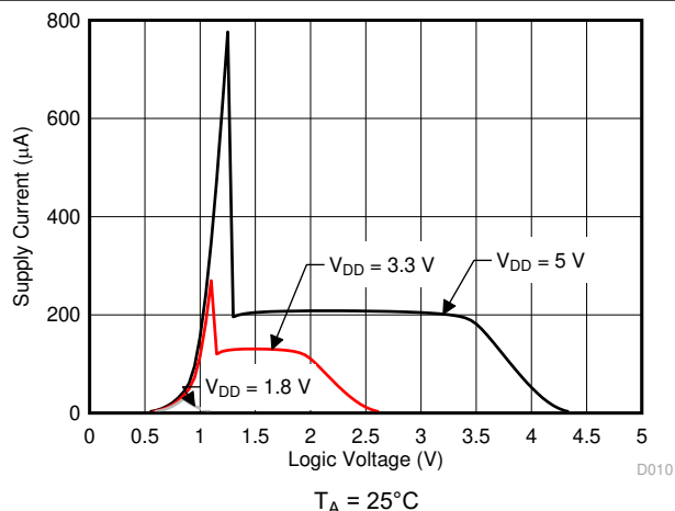
图 5-10. 电源电流与逻辑电压间的关系
