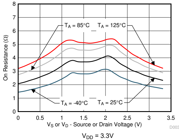
图 5-3. 导通电阻与温度间的关系
