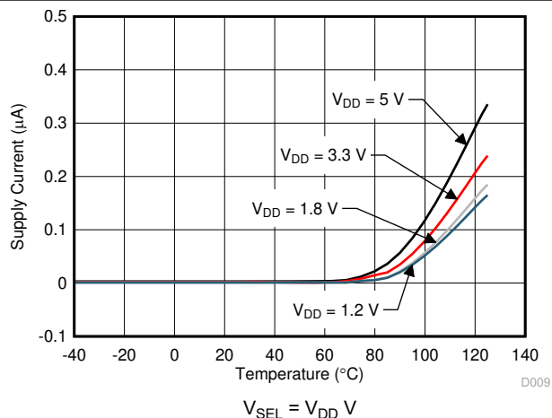
图 5-9. 电源电流与温度间的关系
