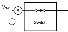
图 7-3. On Leakage
