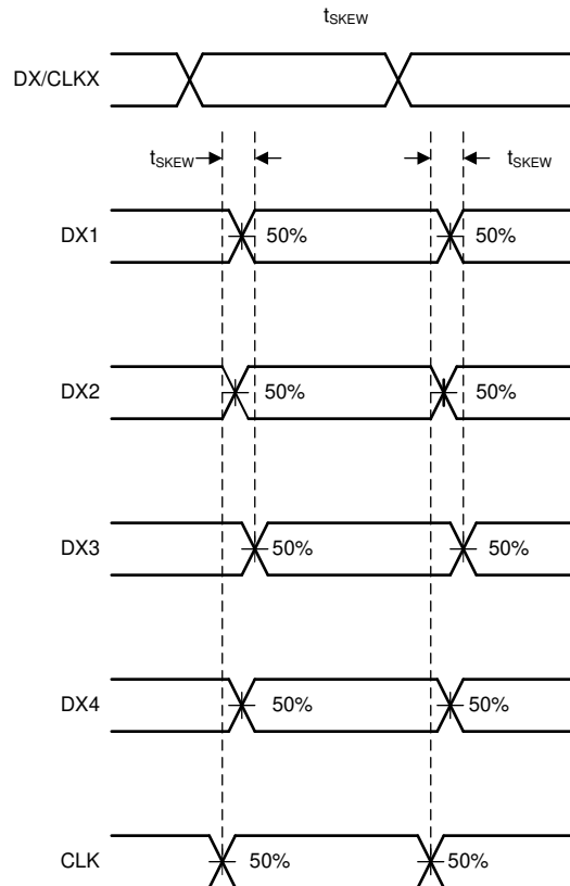
图 7-11. t_{SEW(INTRA)}
