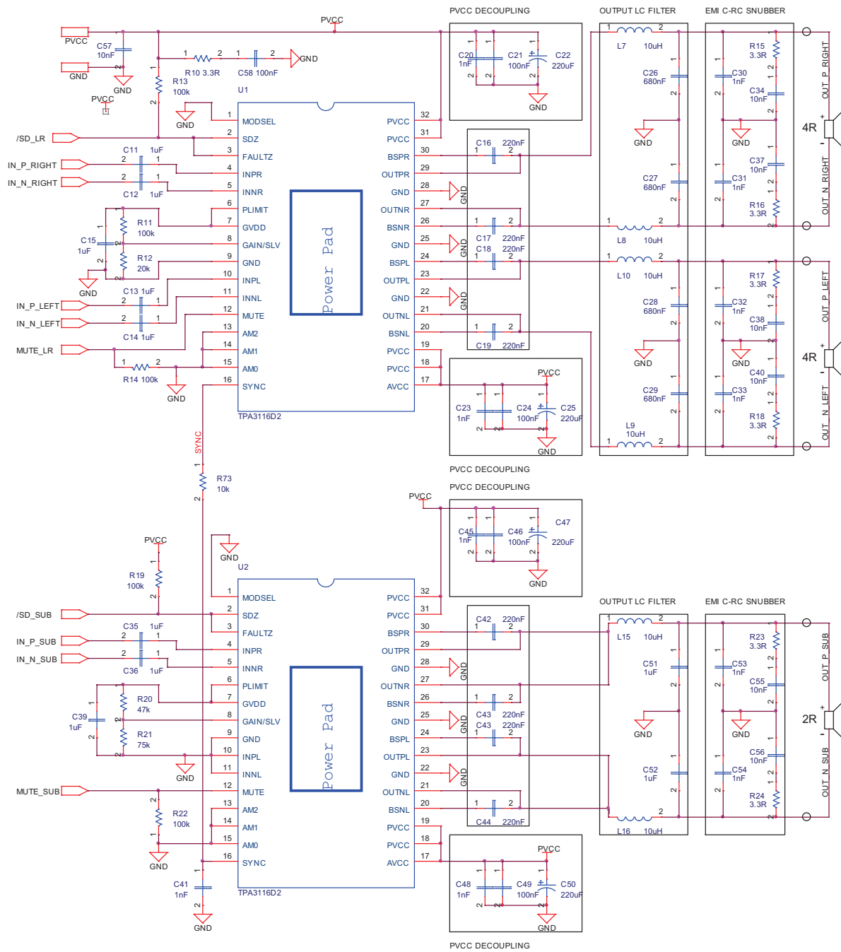
图 37. Schematic
