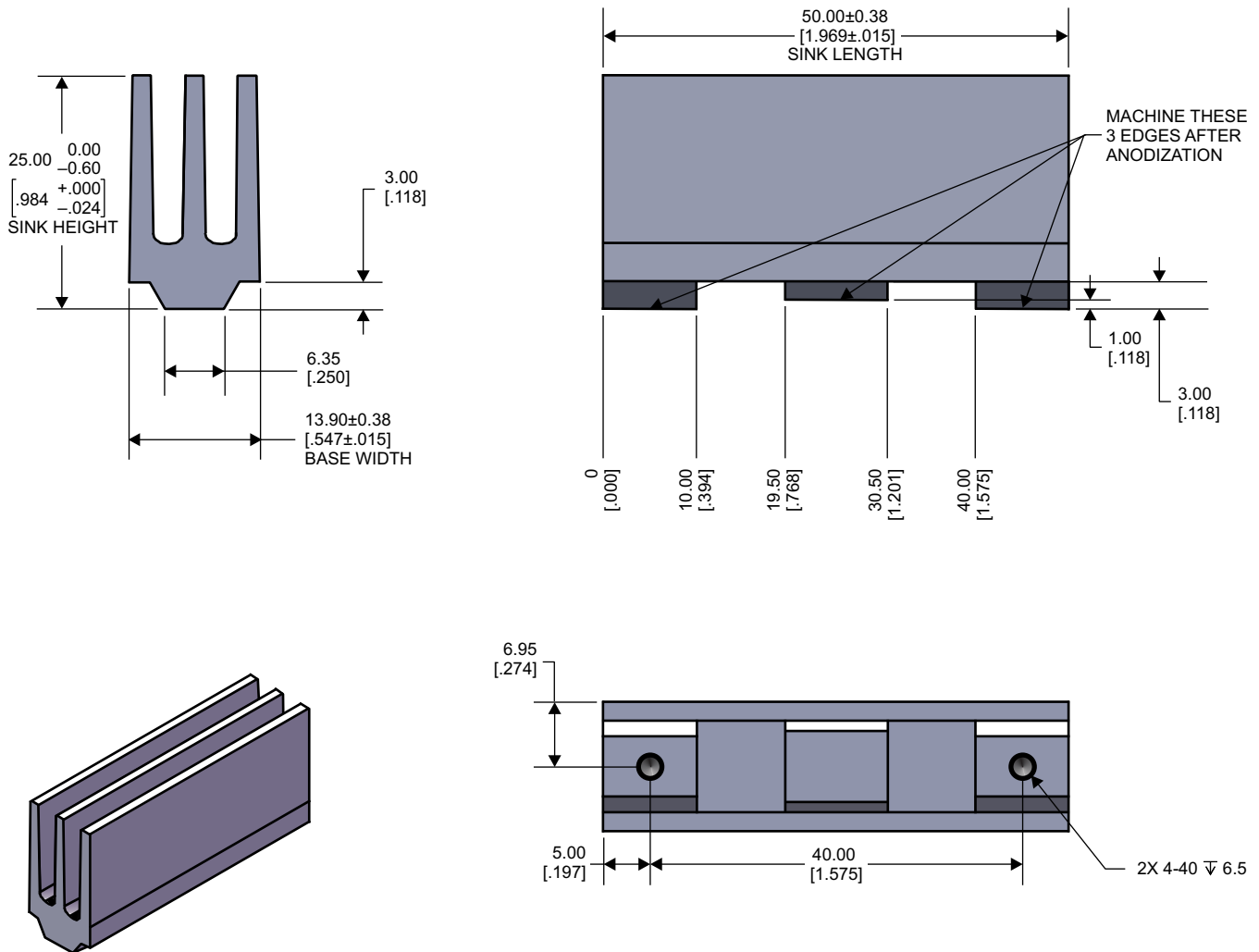
图 42. EVM Heatsink
