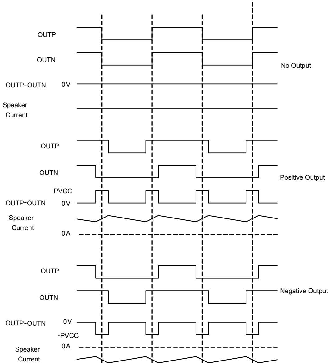
图 7-2. BD Mode Modulation
