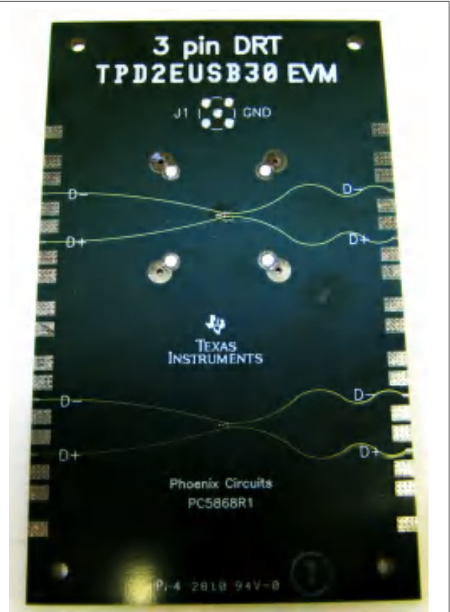
图 10-3. TPDxUSB30/A EVM - TPD2EUSB30/A Side
