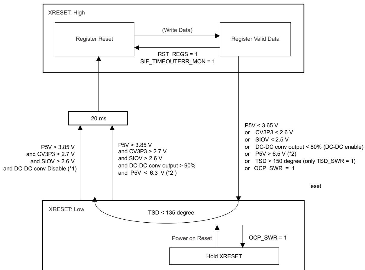
Figure 15. POR Block Diagram
