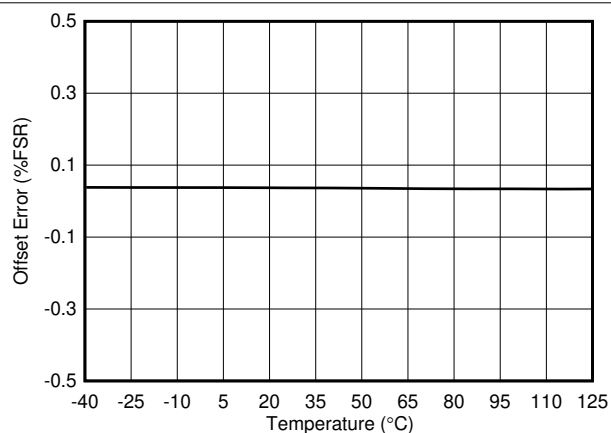
图 6-18. Offset Error vs Temperature
