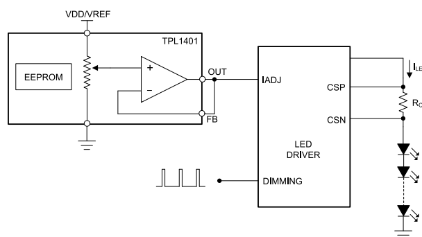
通过 TPL1401 实现可编程电流限制
