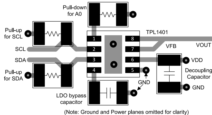
图 10-1. Layout Example
