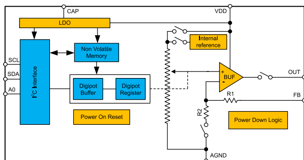
功能方框图
