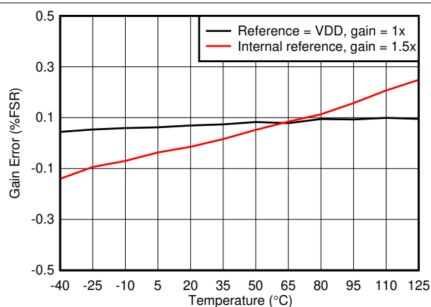
图 6-9. Gain Error vs Temperature
