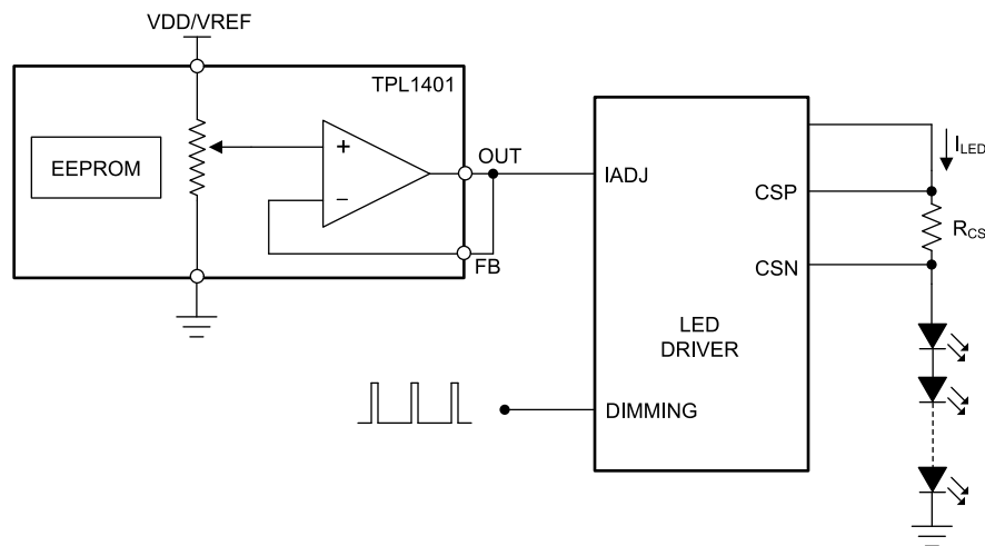
图 8-1. Programmable Current Limit
