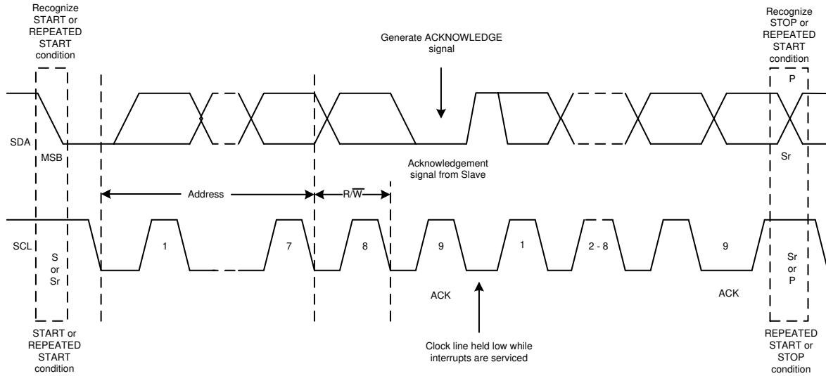
图 7-5. I²C Bus Protocol
