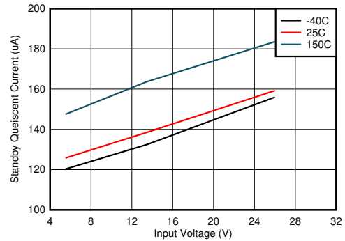
图 8-2. Standby Quiescent Current
