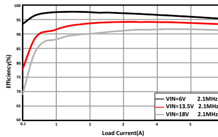
效率与输出电流间的关系
