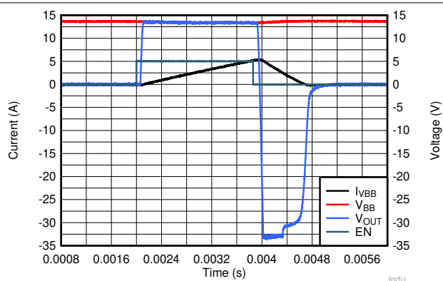
图 7-33. Inductive Load Demagnetization
