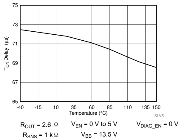
图 7-7. Turn-on Delay Time ( t_{DR} ) vs Temperature
