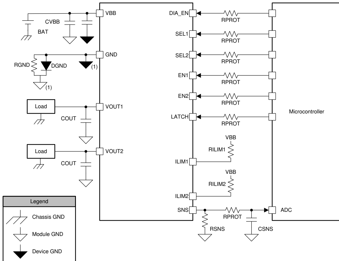
图 15. System Diagram
