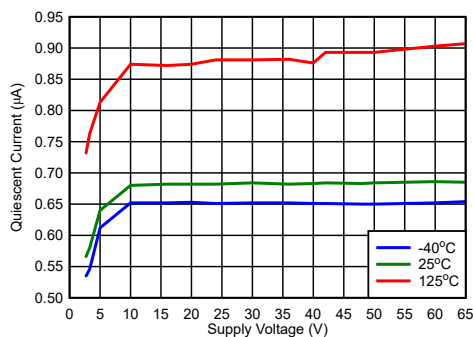
典型 I_{DD} 与 V_{DD}
