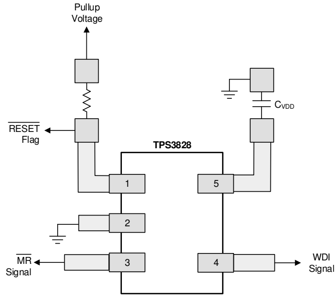
图 8-5. 示例布局 (DBV 封装)
