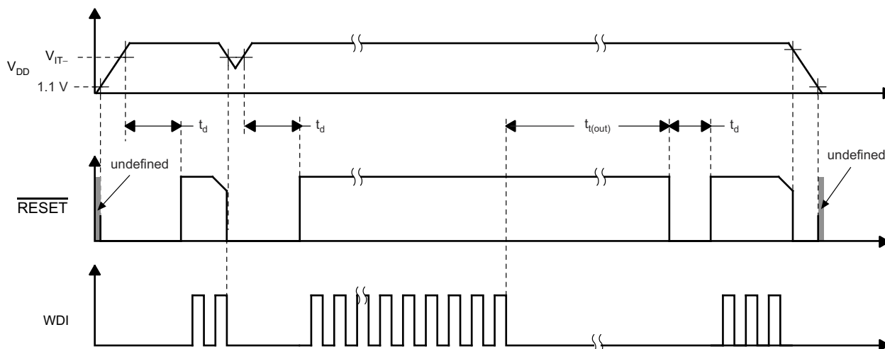
图 6-1. 时序图
