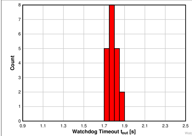
图 6-14. TPS3823A-33 器件在 125°C 时的看门狗超时直方图 (单位数 = 20)
