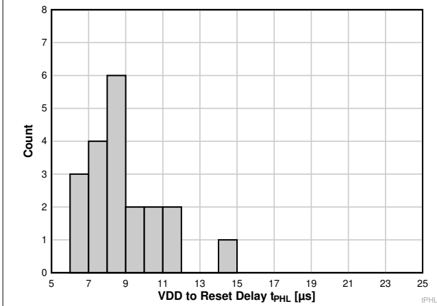
图 6-16. TPS3823A-33 器件在 25°C 时的 VDD 至复位延时直方图 (单位数 = 20)
