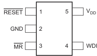
图 5-1. 5 引脚 SOT-23 TPS3820、TPS3823、TPS3823A、TPS3828 : DBV 封装 ( 顶视图 )
