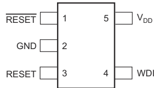
图 5-2. 5 引脚 SOT-23 TPS3824 : DBV 封装 ( 顶视图 )
