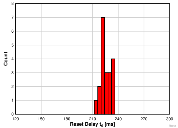
图 6-11. TPS3823A-33 器件在 125^{\circ}\text{C} 时的复位延时直方图 (单位数 = 20)
