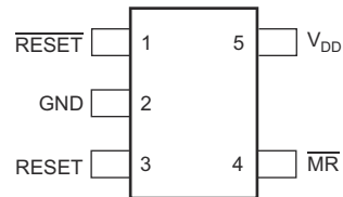
图 5-3. 5 引脚 SOT-23 TPS3825 : DBV 封装 ( 顶视图 )
