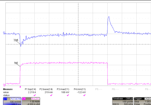
图 22. Load Step Buck 3
