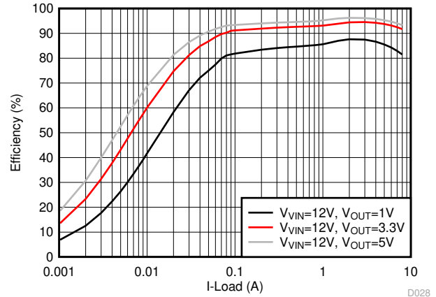
图 6-14. Efficiency, OOA-mode, F_{SW} = 600 kHz
