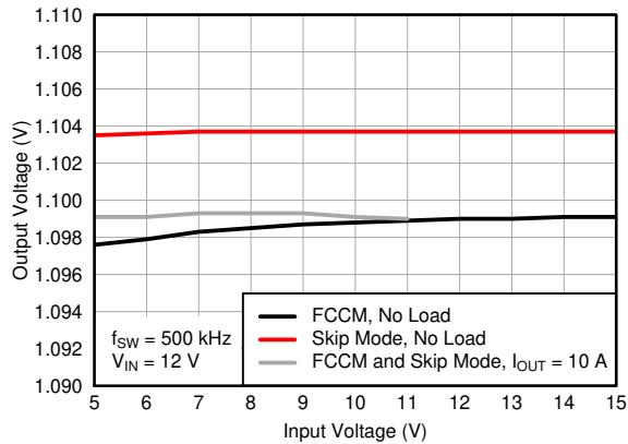
图 5-11. Output Voltage vs Input Voltage
