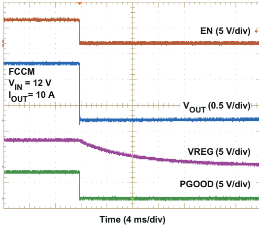
图 7-7. Turn-Off
