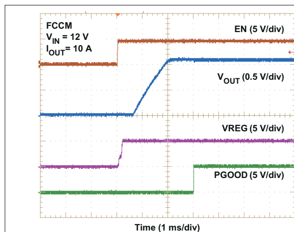
图 7-2. Start-Up
