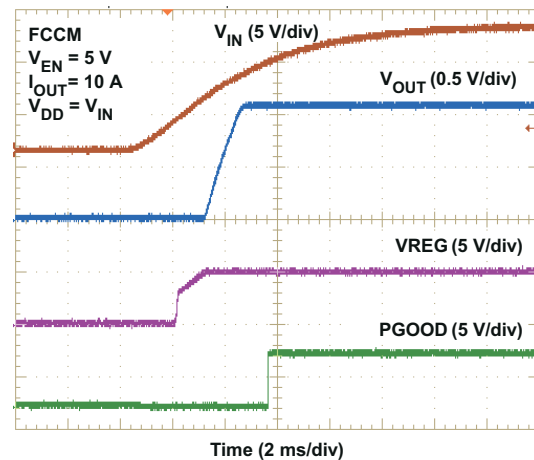
图 7-8. UVLO Start-Up
