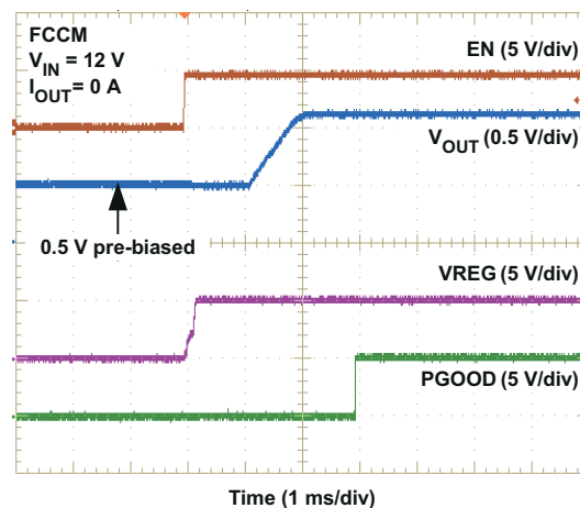
图 7-3. Prebias Start-Up
