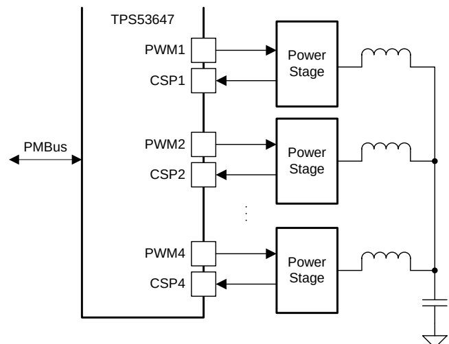
简化原理图
