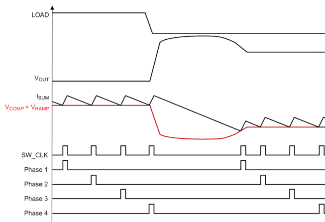
图 11. Load Release
