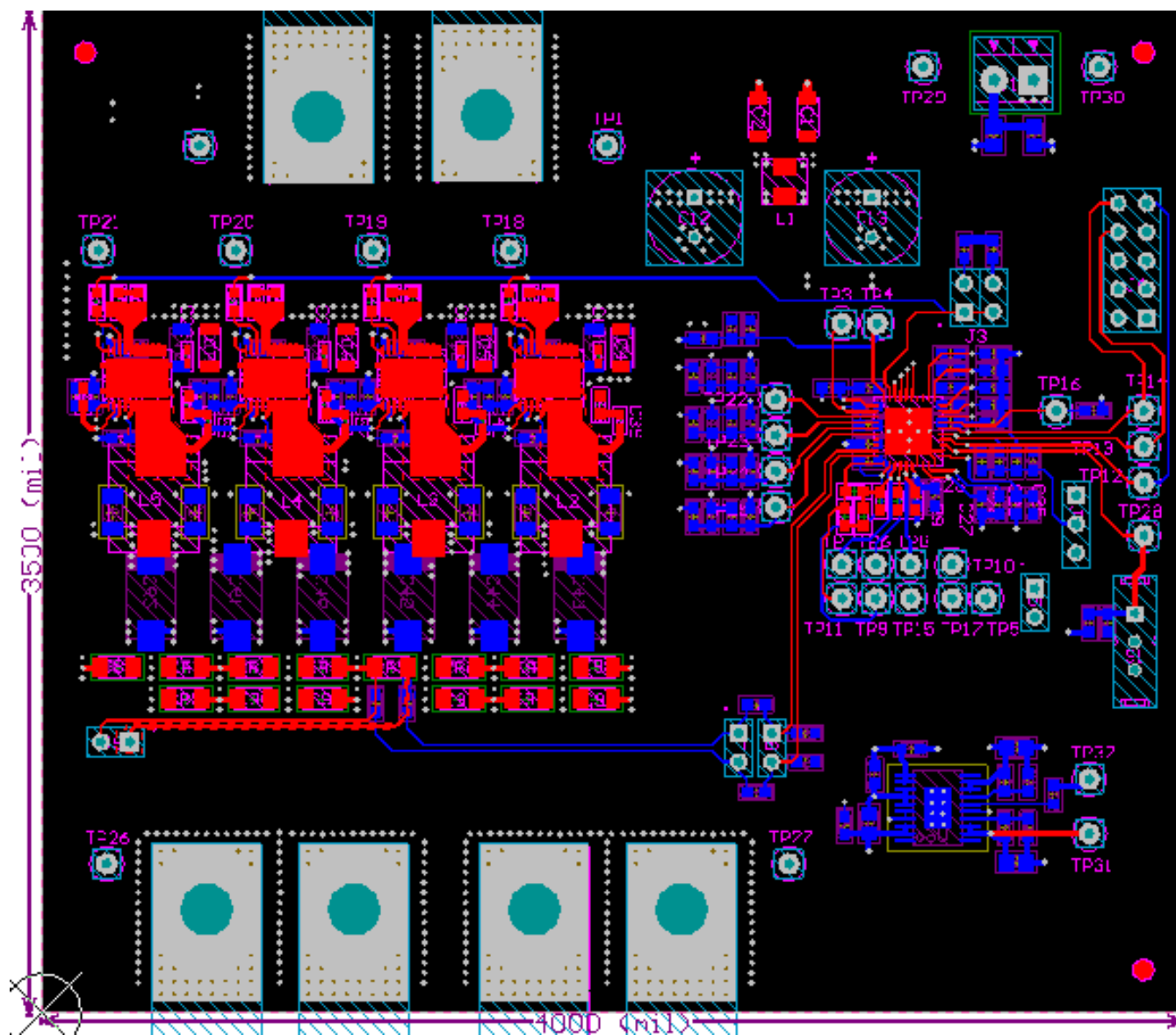
图 124. TPS53647 Layout Example
