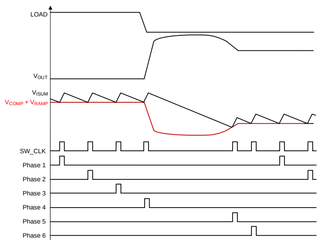
图 11. Load Release
