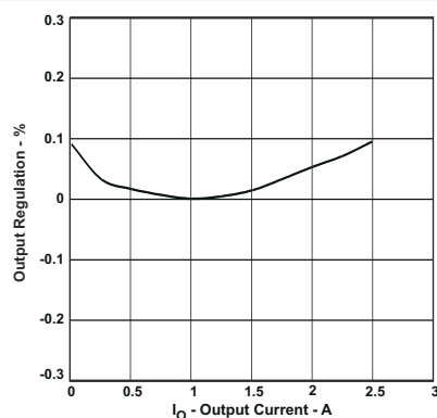
图 7-3. 输出调节百分比与输出电流间的关系
