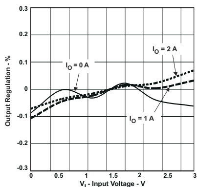
图 7-4. 输入调节百分比与输入电压间的关系
