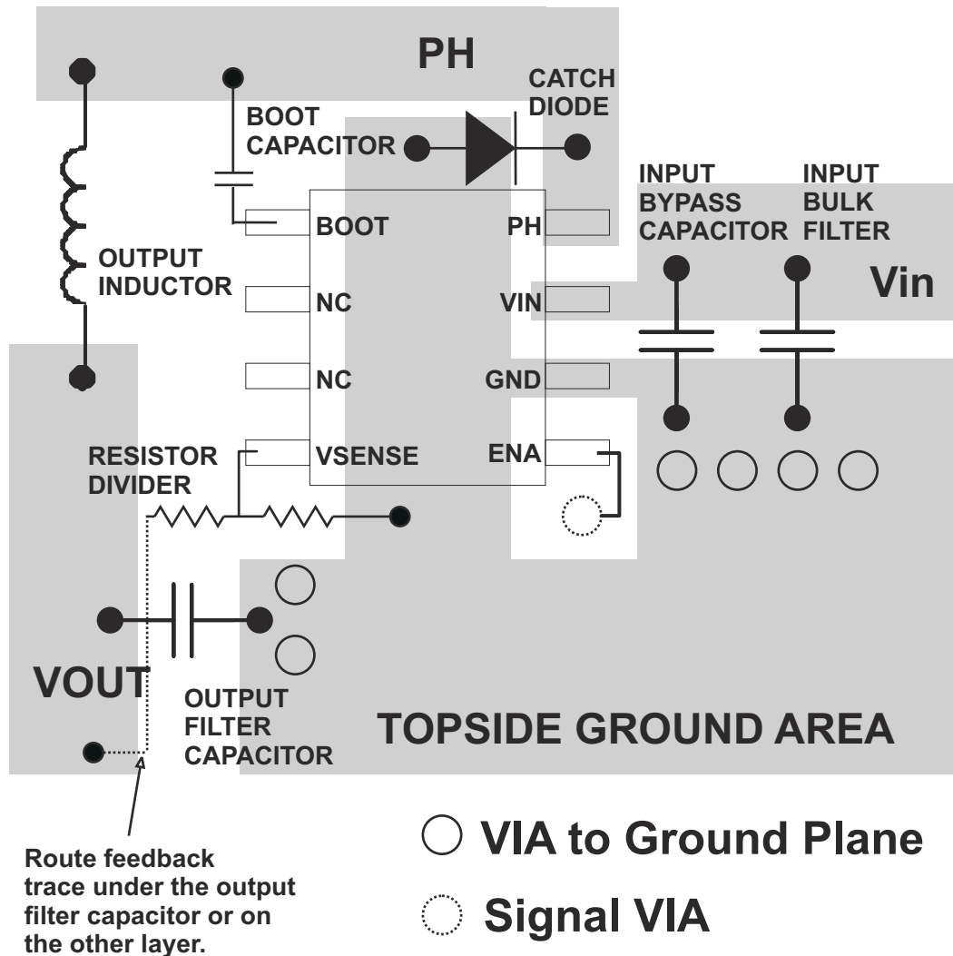
图 7-12. 设计布局
