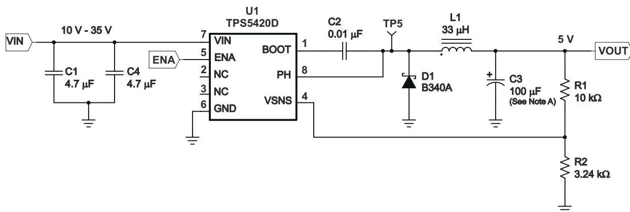
图 7-1. 应用电路，10V — 35V 至 5V
