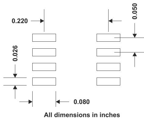
图 7-13. TPS5420 焊盘图案
