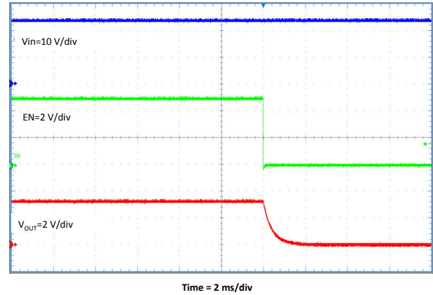
图 7-15. 相对于 EN 的关断
