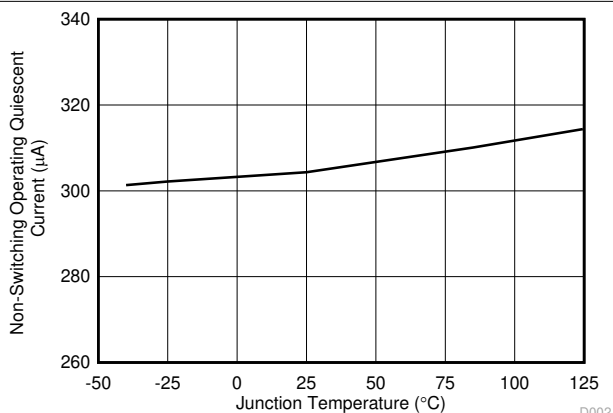
图 5-2. 非开关工作静态电流与结温间的关系
