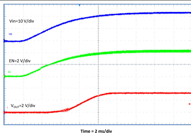
图 7-12. 相对于 VIN 的启动
