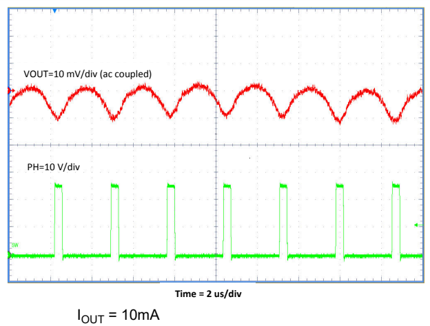
图 7-7. 输出电压纹波
