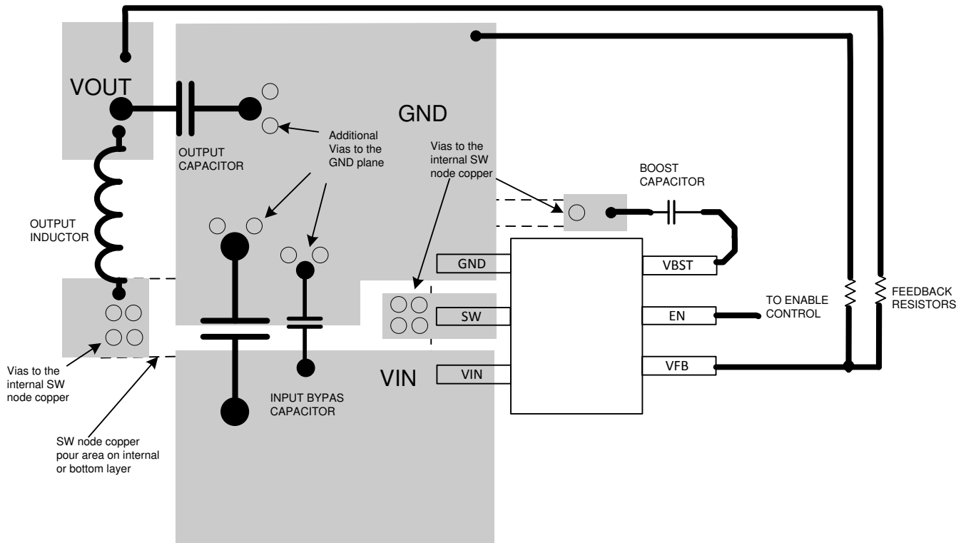
图 7-16. 电路板布局
