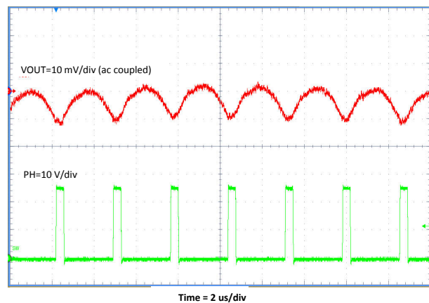
图 7-8. 输出电压纹波
