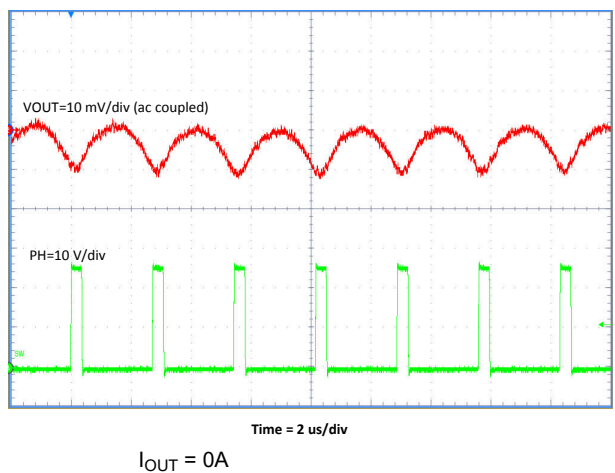
图 7-6. 输出电压纹波
