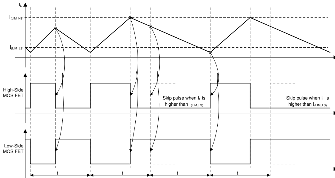
图 6-2. 针对两个 MOSFET 的过流保护
