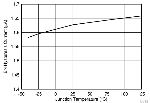
图 5-12. EN 迟滞电流与结温间的关系
