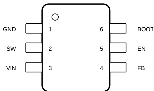
图 4-1.6 引脚 SOT-23-THN , DDC 封装 ( 俯视图 )
