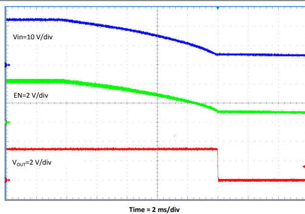
图 7-13. 相对于 VIN 的关断
