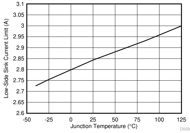
图 5-9. 低侧灌电流限制阈值与结温间的关系
