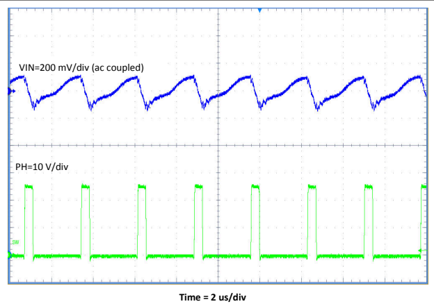
图 7-5. 输入电压纹波
