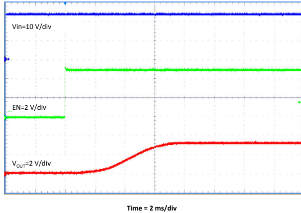
图 7-14. 相对于 EN 的启动
