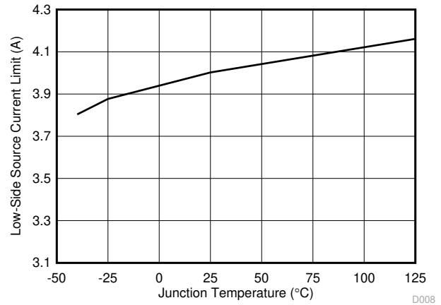
图 5-8. 低侧拉电流限制阈值与结温间的关系
