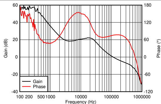
图 8-34. Bode Plot
