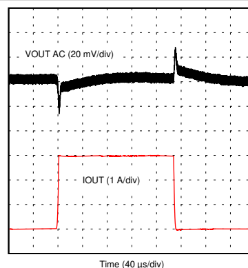
图 8-25. Load Transient
