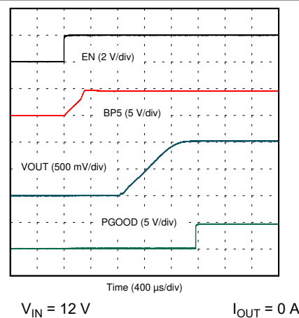
图 8-9. EN Start-up – Measuring BP5
