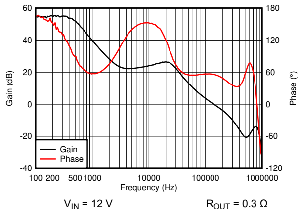
图 8-7. Bode Plot
