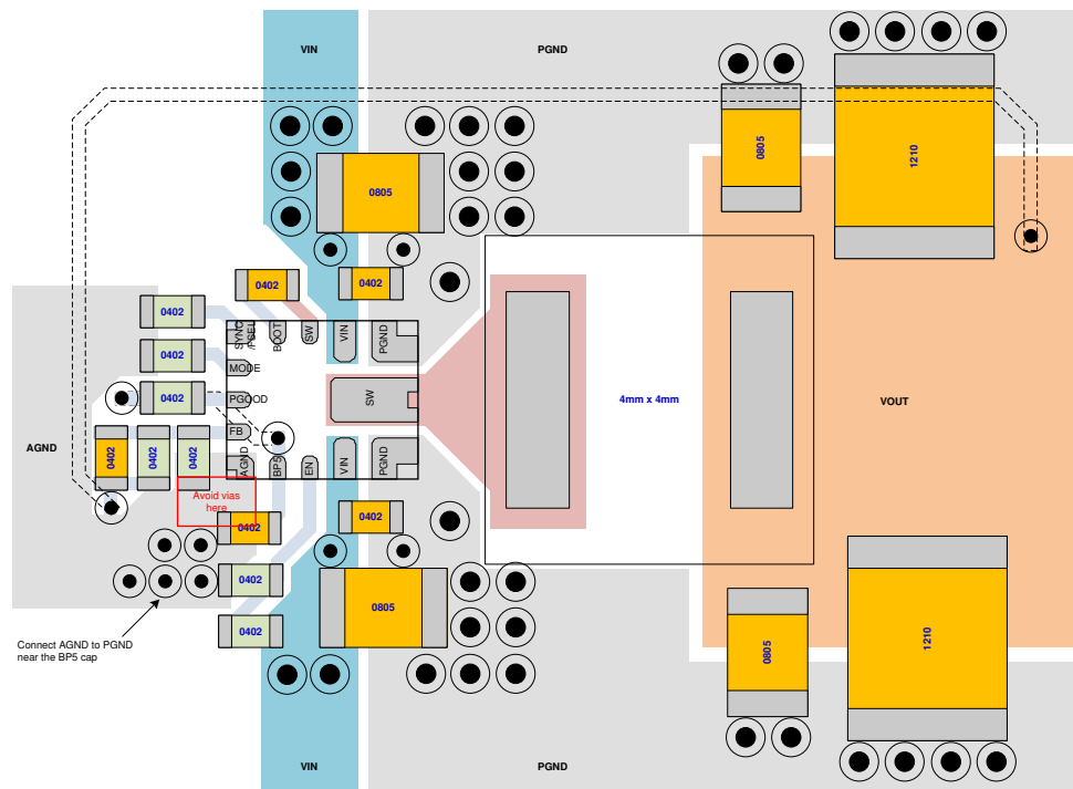
图 10-1. Example PCB Layout
