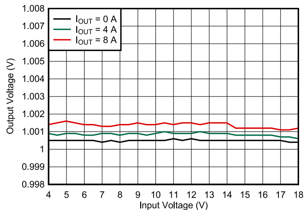
图 8-6. Line Regulation
