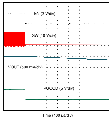
图 8-11. EN Shutdown
