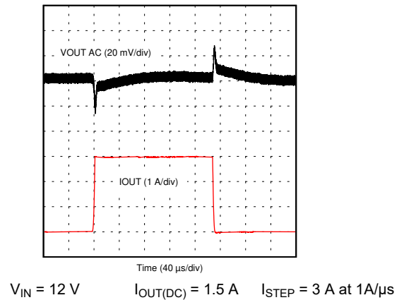
图 8-25. Load Transient
