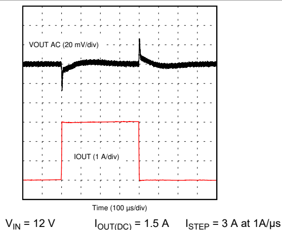
图 8-8. Load Transient
