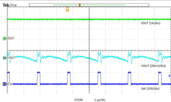
图 8-23. Output Voltage Ripple, FCCM, 20-A Load
