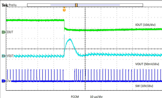
图 6-12. Unload Transient
