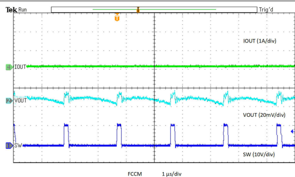
图 8-21. Output Voltage Ripple, FCCM, 0-A Load
