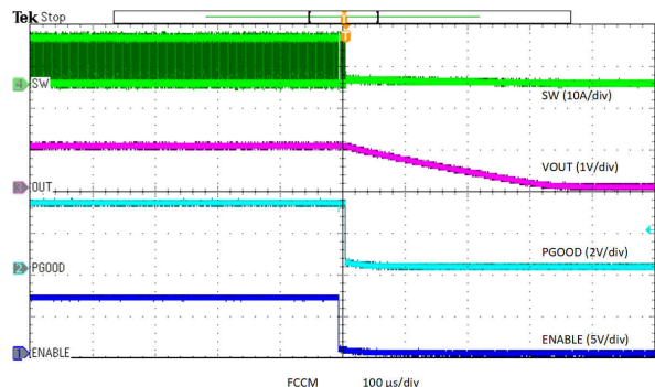
图 8-15. Prebias Power Down
