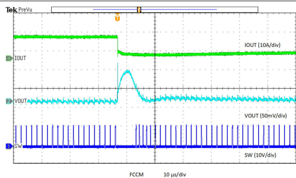
图 8-20. Unload Transient
