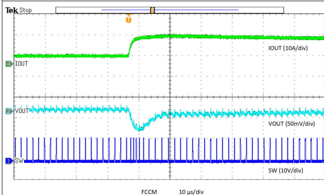
图 6-11. Load Transient
