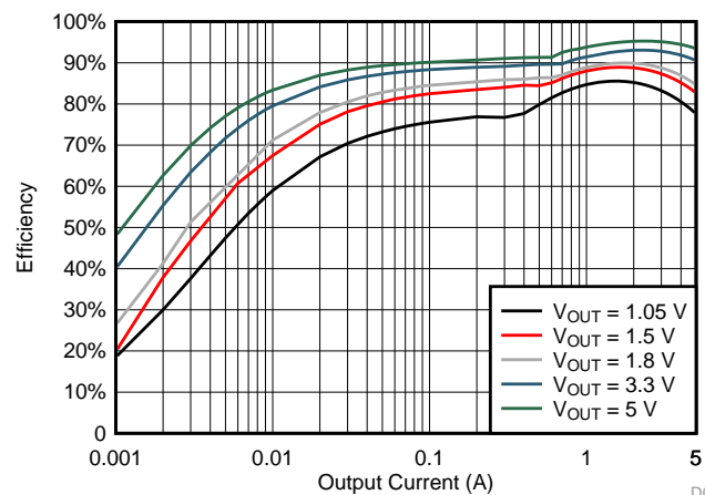
TPS565201 效率
